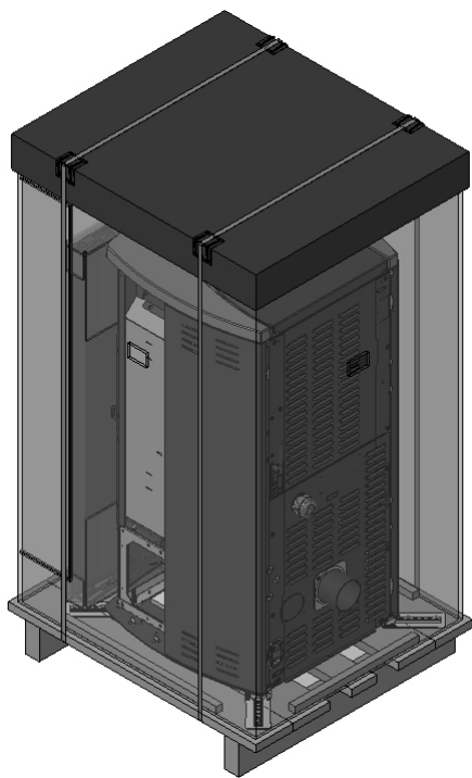
OPAKOWANIE EGO ZE STALOWĄ POWŁOKĄ
