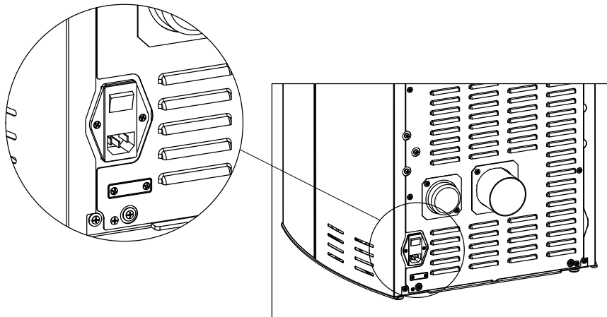
POŁĄCZENIE ELEKTRYCZNE PIECA
