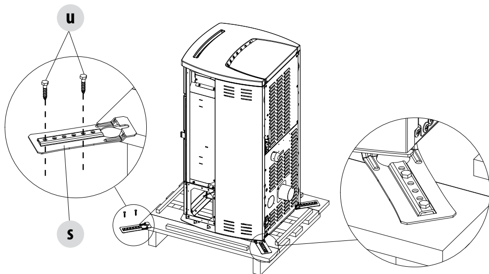
ZDJĘCIE UCHWYTÓW MOCUJĄCYCH (NA RYSUNKI PIEC EGO)
