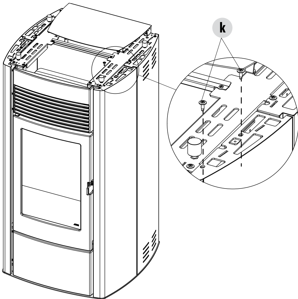
MOCOWANIE GÓRNEJ METALOWEJ PŁYTY
