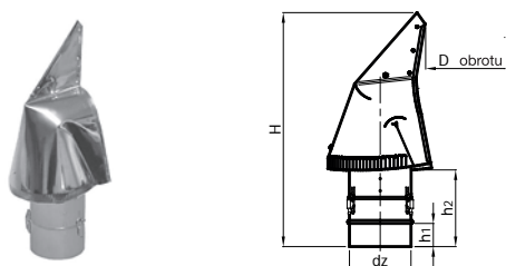
8. Podstawa rurowa otwierana Ø150÷Ø300 -B
