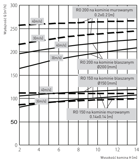
Wykres wydajności samonastawnych nasad kominowych ROTOWENT Ø150 i Ø200 dla kominu blaszanego i murowanego, dla dwóch prędkości wiatru 3 i 4 [m/s].
