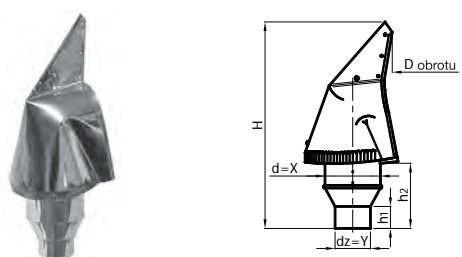
10. Podstawa redukcyjna -X/Y-...-B-S
