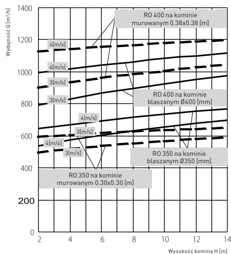
Wykres wydajności samonastawnych nasad kominowych ROTOWENT Ø350 i Ø400 dla kominu blaszanego i murowanego, dla dwóch prędkości wiatru 3 i 4 [m/s].
