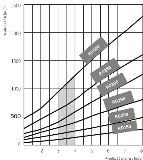
Wykres wydajności samonastawnych nasad kominowych ROTOWENT w zależności od prędkości wiejącego wiatru bez uwzględnienia wysokości kominu.
