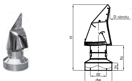
6. Podstawa z kołnierzem zamykającym ocieplenie otwierana -B-K-U
