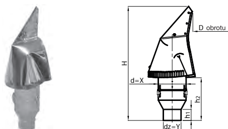
11. Podstawa redukcyjna otwierana Ø150÷Ø300 -X/Y-...-B
