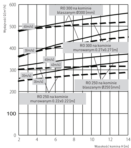
Wykres wydajności samonastawnych nasad kominowych ROTOWENT Ø250 i Ø300 dla kominu blaszanego i murowanego, dla dwóch prędkości wiatru 3 i 4 [m/s].
