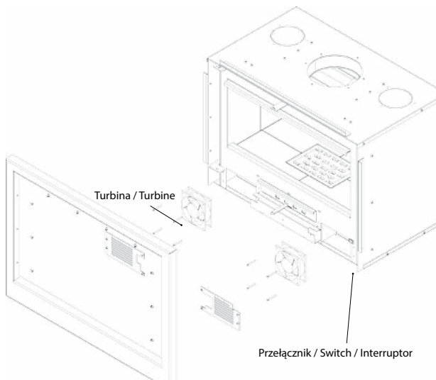
Rys. 2. Kasetka ARKE – sposób montażu wentylatorów wraz z umiejscowieniem przełącznika
