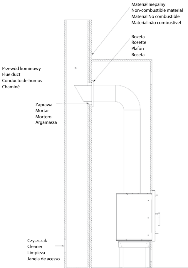
Rys. 4. Kasetta ARKE – przykładowe podłączenie do komina Fig. 4. ARKE cassette - exemplary connection to the chimney Fig. 4. Cassete ARKE . Ejemplo de conexión a la chimenea Fig. 4 - recuperador de calor ARKE - exemplo de ligação à chaminé
