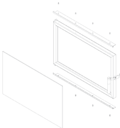
Rys. 6. Kasetta ARKE - demontaż szyby
