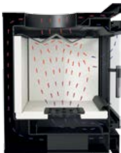
Rys. 1. Kasetka ARKE – obieg powietrza we wkładzie kominkowym ARKE
