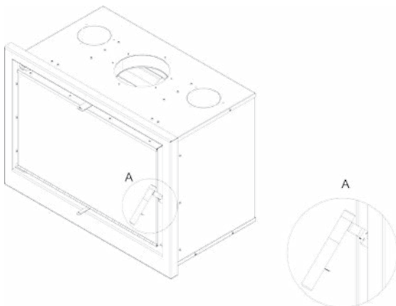
Rys. 8. Kaseta ARKE – demontaż drzwi krok 2
