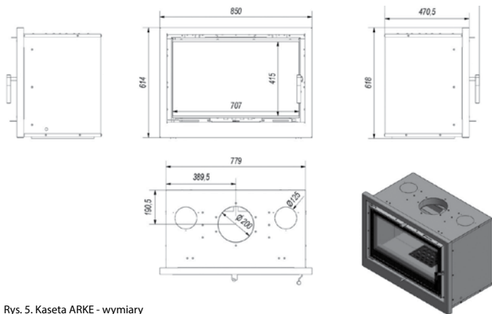
Rys. 5. Kasetta ARKE - wymiary
