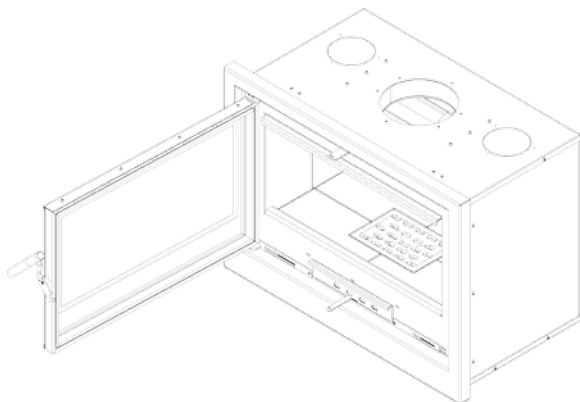
Rys. 9. Kaseta ARKE – demontaż drzwi krok 3
