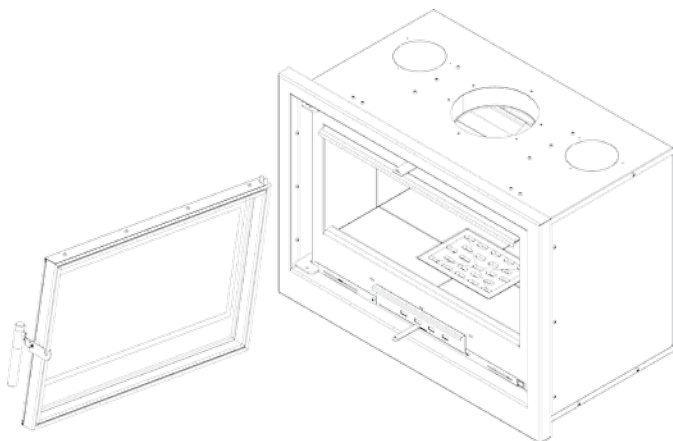
Rys. 12. Kaseta ARKE – demontaż drzwi krok 6
