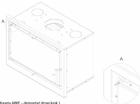
Rys. 7. Kaseta ARKE – demontaż drzwi krok 1
