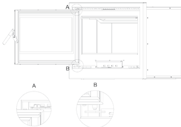
Rys. 10. Kaseta ARKE – demontaż drzwi krok 4
