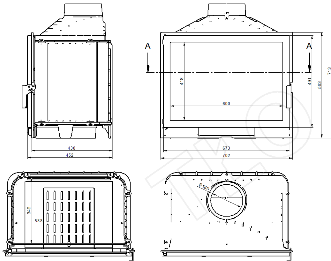
SECTION A-A
