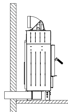
Rysunek 18. Podłączenie wkładu kominkowego do zewnętrznego wlotu powietrza.
