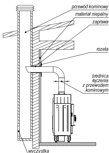
Rysunek 19. Podłączenie wkładu kominkowego do przewodu kominowego.
