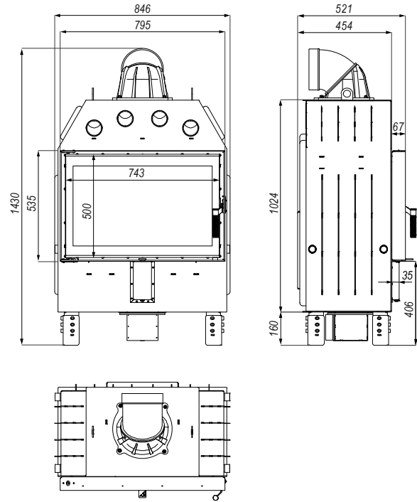
Rysunek 6. Wymiary wkładu kominkowego PRIMA ME.
