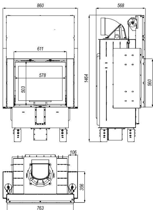
Rysunek 8. Wymiary wkładu kominkowego PRIMA SM G.
