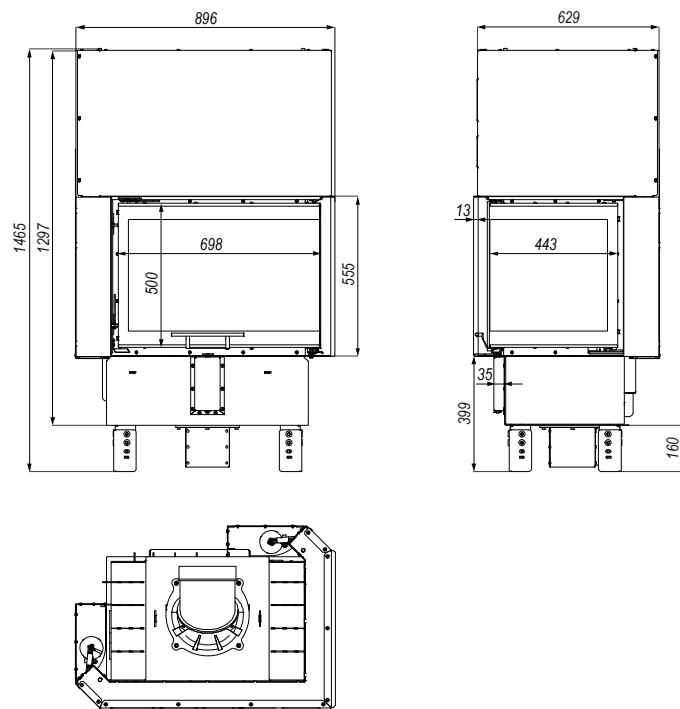
Rysunek 14. Wymiary wkładu kominkowego PRIMA SM BP G.
