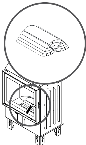
Rysunek 21. Sposób ułożenia paliwa podczas rozpalania.
