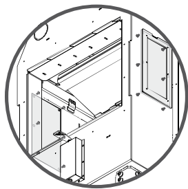
Rysunek 27. Demontaż pokryw otworów rewizyjnych w bocznych ścianach wkładu PRIMA wersji G.
