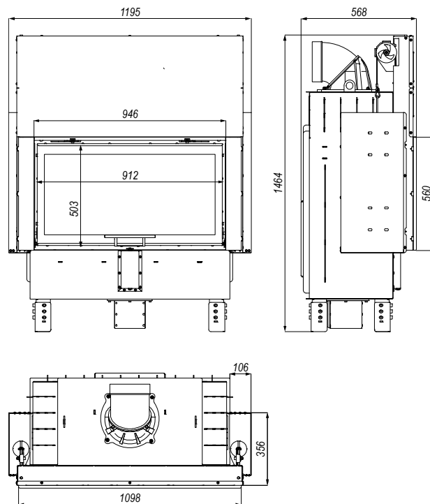
Rysunek 10. Wymiary wkładu kominkowego PRIMA LA G.
