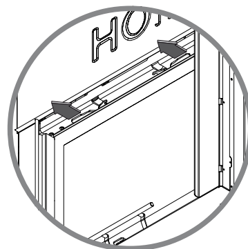
Rysunek 22. Umieszczenie rygli pozwalających na otwarcie drzwi w pozycji uchylniej w PRIMA G.
