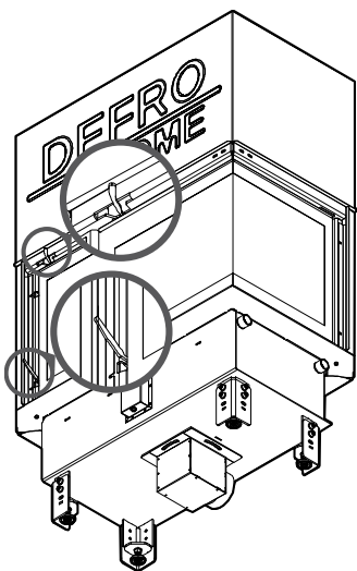
Rysunek 24. Umieszczenie rygli pozwalających na otwarcie drzwi w pozycji uchylnej w PRIMA BP G.
