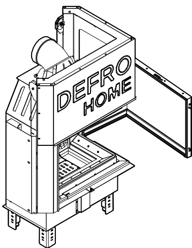
Rysunek 25. Widok kominka z szybą boczną i drzwiami gilotynowymi w pozycji uchylnej.
