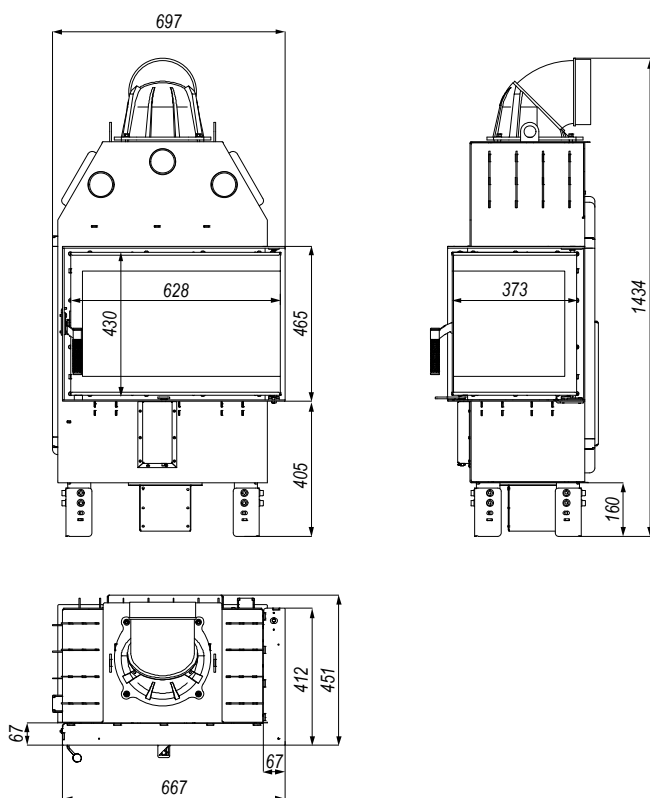
Rysunek 13. Wymiary wkładu kominkowego PRIMA SM BP MINI.
