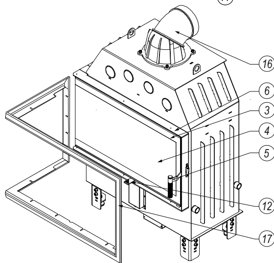
Rysunek 3. Budowa wkładu kominkowego PRIMA z szybą boczną. 1 – korpus, 2 – komora paleniskowa, 3 – drzwi, 4 – szyba żaroodporna, 5 – klamka z rygłem, 6 – ramka futryny, 7 – podłoga, 8 – ruszt, 9 – pojemnik popielnika, 10 – króciec poboru powietrza, 11 – regulacja dopływu powietrza, 12 – suwak regulacji dopływu powietrza, 13 – okładziny z betonu żaroodpornego, 14 – otwory z systemu dopalenia spalin, 15 – deflektor, 16 – czopuch, 17 – maskownica.
