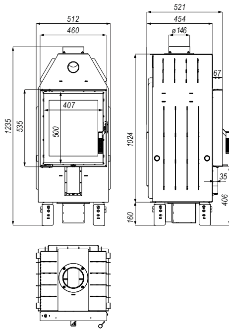
Rysunek 4. Wymiary wkładu kominkowego PRIMA XSM.
