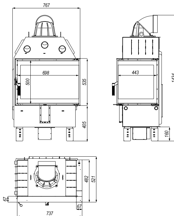
Rysunek 11. Wymiary wkładu kominkowego PRIMA SM BP.
