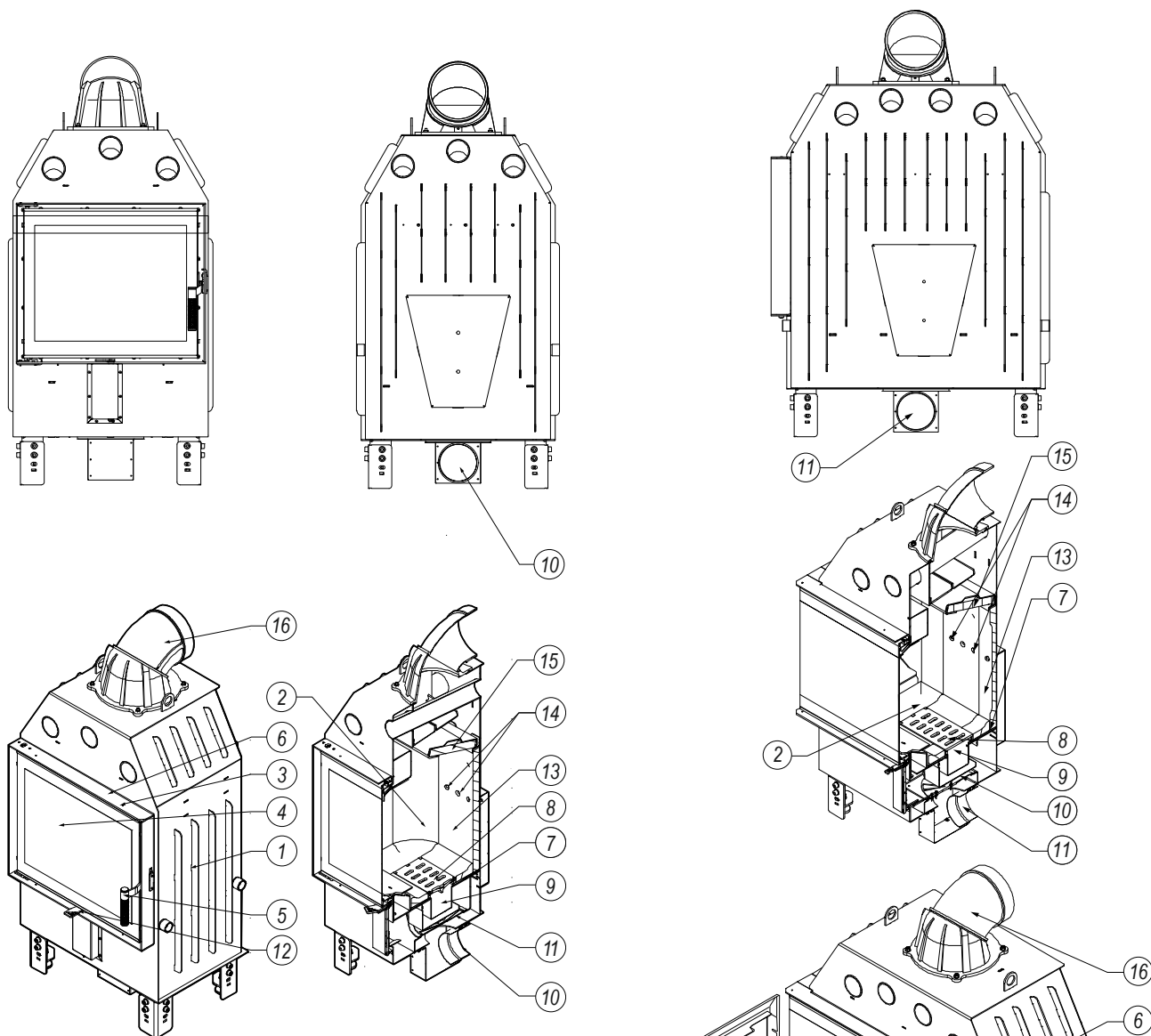
Rysunek 2. Budowa wkładu kominkowego PRIMA w wersji podstawowej.
