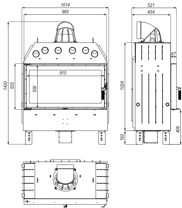
Rysunek 7. Wymiary wkładu kominkowego PRIMA LA.
