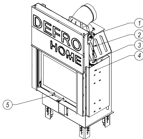
Rysunek 1. Budowa wkładu kominkowego PRIMA w wersji G.
