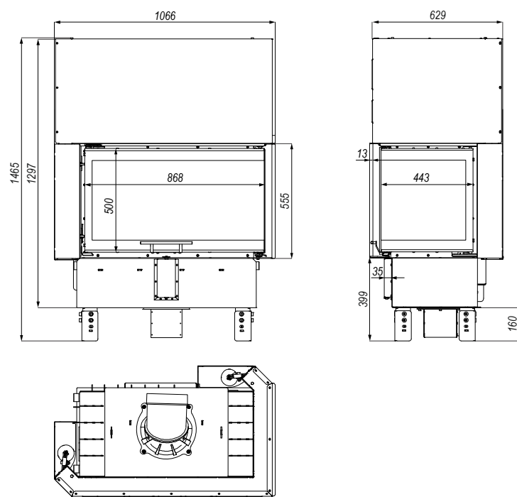
Rysunek 15. Wymiary wkładu kominkowego PRIMA ME BP G.
