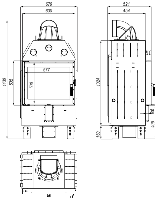
Rysunek 5. Wymiary wkładu kominkowego PRIMA SM.
