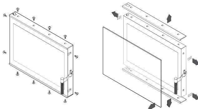
Rysunek 26. Demontaż szyby w drzwiach.
