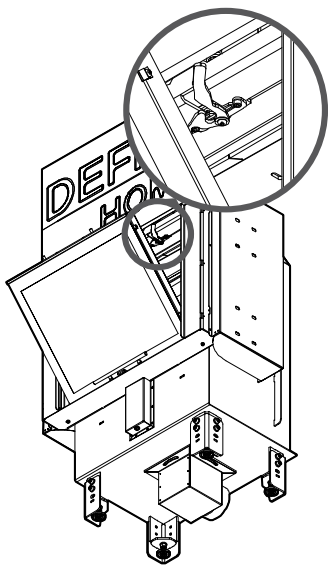
Rysunek 23. Widok wkładu kominkowego PRIMA G z drzwiami w pozycji uchylnej.
