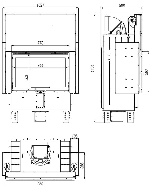
Rysunek 9. Wymiary wkładu kominkowego PRIMA ME G.
