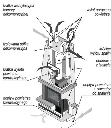
Rysunek 17. System dystrybucji gorącego powietrza.
