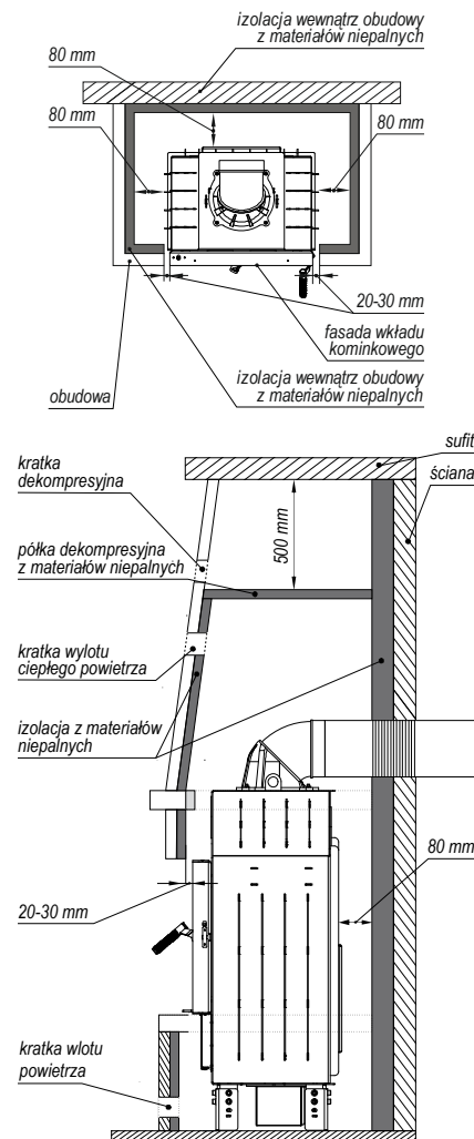
Rysunek 16. Przykładowa zabudowa wkładu kominkowego.
