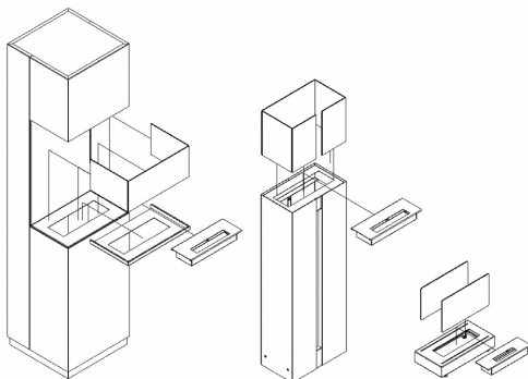
Fig. 5. Metodo di montaggio dei vetri nei biocaminetti Sierra, Romeo, Galina
