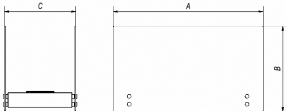
Obr. 8: Způsob dimenzování biokrbů Foxtrot, Galina, Hotel, Hotel Mini, Hotel Krzak, Hotel Mini Krzak, Linate
