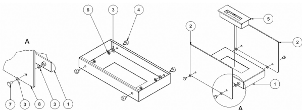
Dibujó 3. Modo de instalación de biochimeneas: Hotel, Mini, Bush Hotel, Hotel Mini Busch
