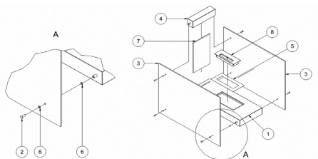
4.sz.kép: Linatite bio kandalló szerelésének módja
