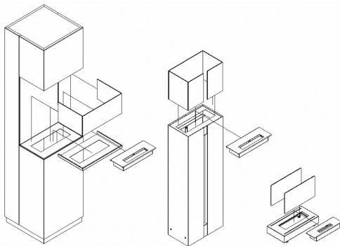
5.sz.kép: A Sierra, Romeo, Galina bio kandallók üvegei szerelésének módja
