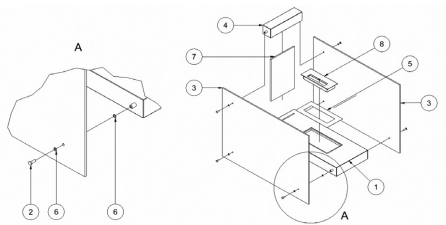
Slika 4. Način montaže bio-kamina Liniate
