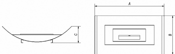
Εικ. 8 Τρόπος μέτρησης διαστάσεων των βιολογικών τζακιών „India Mini“, „India Max“, „Kilo“, „Misa“, „Misa Mini“
