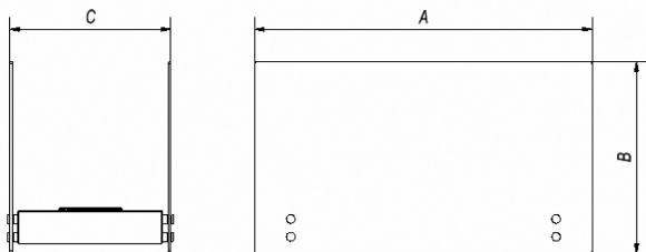
Dessin 8. Manière de mesurer les bio-cheminées „Foxtroł“, „Galina“, „Hotel“, „Hotel Mini“, „Hotel Krzak“, „Hotel Mini Krzak“, „Linate“ matavimo būdas
