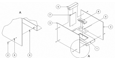
Dibujó 4. Modo de instalación de biochimenea Linate
