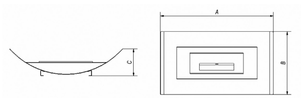
Obr. 9: Způsob dimenzování biokrbů India, India Mini, India Max, Kilo, Misa, Misa Mini
