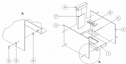
4. attēls. Stikla montāža biokamīnos Linate
