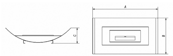
Obr. 9: Spôsob dimenzovania biokozubov India, India Mini, India Max, Kilo, Misa, Misa Mini
