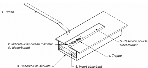
Dessin 2. Bio-bloc de combustion – vue en coupe
