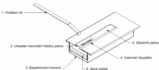
Obr. 2: Nádobna na biopalivo – průřez
