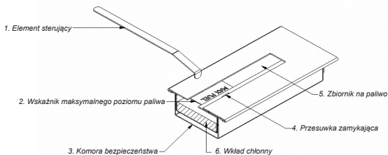
Rys. 2. Biopojemnik - przekrój
