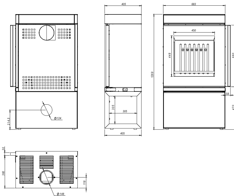
Rysunek 2. Wymiary pieca wolnostojącego CUBE.
