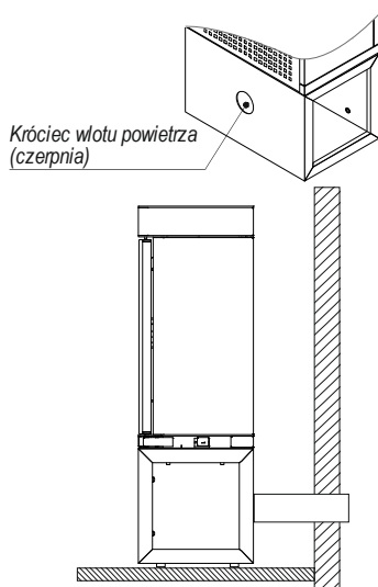
Rysunek 4. Podłączenie pieca wolnostojącego CUBE do zewnętrznego wlotu powietrza.
