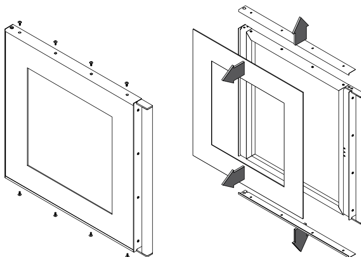
Rysunek 8. Demontaż szyby w drzwiach.
