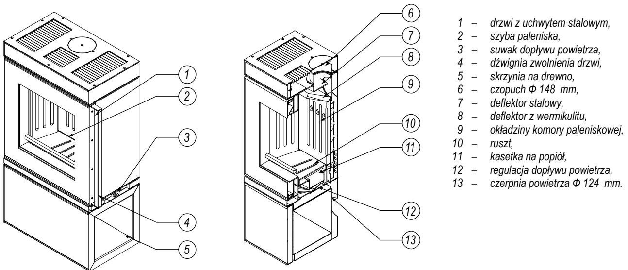
Rysunek 1. Budowa pieca wolnostojącego CUBE.
