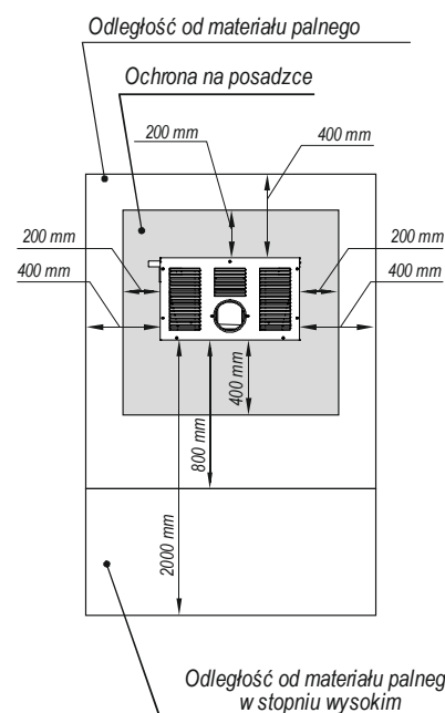
Rysunek 3. Minimalne bezpieczne odległości przy ustawianiu pieca wolnostojącego.
