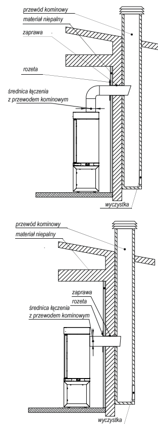
Rysunek 5. Możliwości podłączenie pieca kominowego do przewodu kominowego
