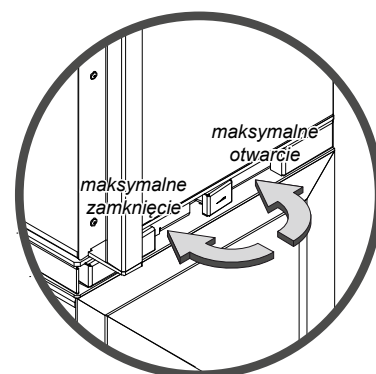
Rysunek 6. Ustawienie suwaka regulacji dopływu powietrza
