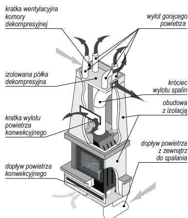
Rysunek 8. System dystrybucji gorącego powietrza.
