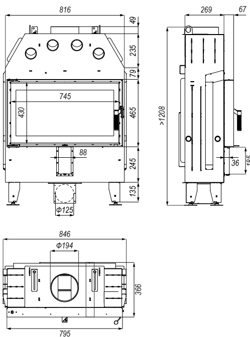
Rysunek 4. Wymiary wkładu kominkowego INTRA ME SLIM.
