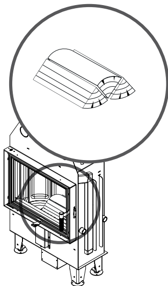
Rysunek 12. Sposób ułożenia paliwa podczas rozpalenia.
