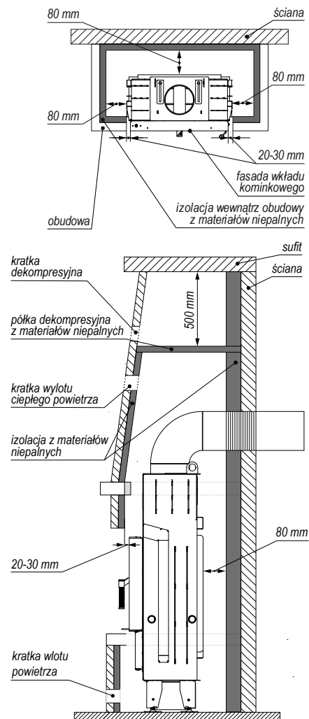
Rysunek 7. Przykładowa zabudowa wkładu kominkowego.
