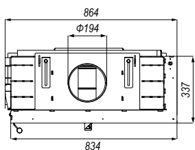
Rysunek 6. Wymiary wkładu kominkowego INTRA ME BP SLIM.
