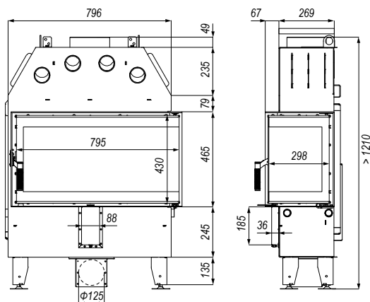
Rysunek 5. Wymiary wkładu kominkowego INTRA SM BP SLIM.
