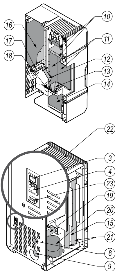
Rysunek 2. Budowa pieca kominkowego OMNIPPELL.
