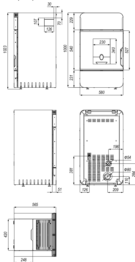
Rysunek 3. Wymiary pieca kominkowego OMNIPPELL.
