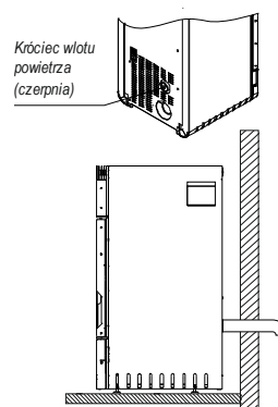
Rysunek 5. Podłączenie pieca kominkowego OMNIPPELL do zewnętrznego wlotu powietrza.
