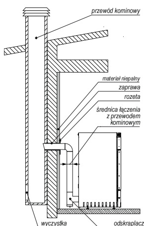
Rysunek 6. Przykład podłączenie pieca OMNIPELL do przewodu kominowego bez odprowadzania skroplin.
