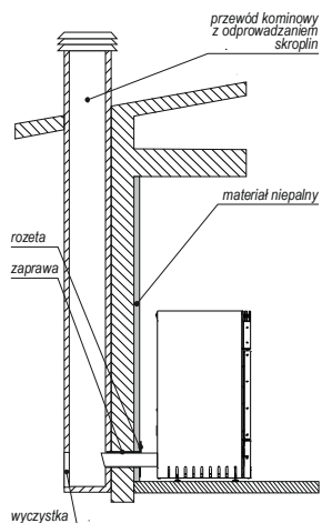
Rysunek 7. Przykład podłączenie pieca OMNIPELL do przewodu kominowego z odprowadzaniem skroplin.
