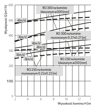
Wykres wydajności samonastawnych nasad kominowych ROTOWENT ø250 i ø300 dla kominu blaszanego i muruwanego, dla dwóch prędkości wiatru 3 i 4 [m/s].
