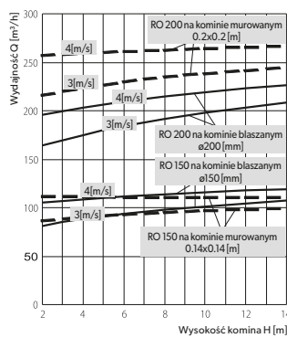
Wykres wydajności samonastawnych nasad kominowych ROTOWENT ø150 i ø200 dla kominu blaszanego i muruwanego, dla dwóch prędkości wiatru 3 i 4 [m/s].
