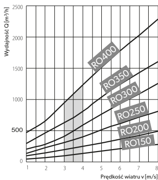
Wykres wydajności samonastawnych nasad kominowych ROTOWENT w zależności od prędkości wiatru bez uwzględnienia wysokości kominu. *1 [m/s] = 3.6 [km/h]
