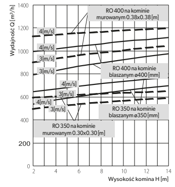
Wykres wydajności samonastawnych nasad kominowych ROTOWENT ø350 i ø400 dla kominu blaszanego i muruwanego, dla dwóch prędkości wiatru 3 i 4 [m/s].
