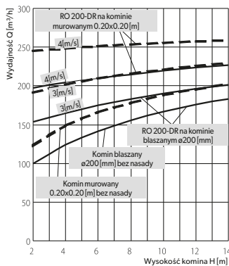
Wykres wydajności samonastawnych nasad kominowych ROTOWENT DRAGON Ø200 dla kominu blaszanego i muranego, dla dwóch prędkości wiatru 3 i 4 [m/s].
