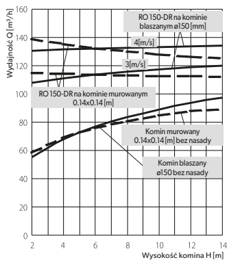
Wykres wydajności samonastawnych nasad kominowych ROTOWENT DRAGON Ø150 dla kominu blaszanego i muranego, dla dwóch prędkości wiatru 3 i 4 [m/s].
