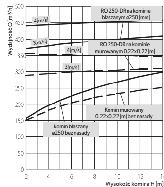
Wykres wydajności samonastawnych nasad kominowych ROTOWENT DRAGON Ø250 dla kominu blaszanego i muranego, dla dwóch prędkości wiatru 3 i 4 [m/s].
