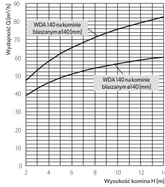
Wykres wydajności daszka wywiewnikowego ø100, 130, 140 dla kominia blaszanego przy zerowej prędkości wiatru.
