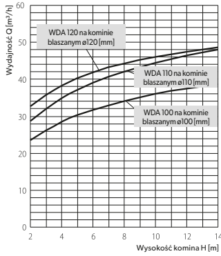
Wykres wydajności daszka wywiewnikowego ø100, 110, 120 dla kominia blaszanego przy zerowej prędkości wiatru.
