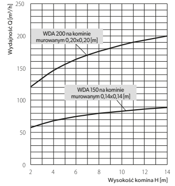
Wykres wydajności daszka wywiewnikowego ø150, 200 dla kominia muranego przy zerowej prędkości wiatru.
