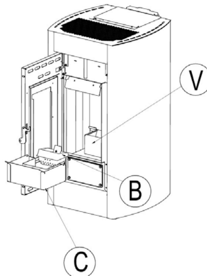
Fig. 33 - Czyszczenie
