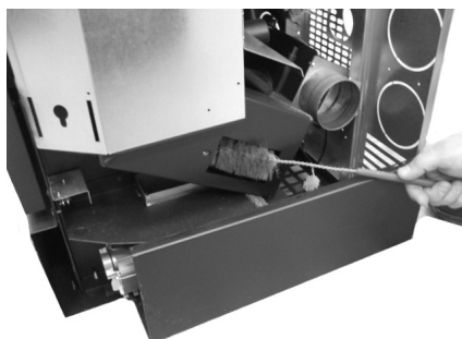
Fig. 100 - Czyszczenie szczotką do rur 2
