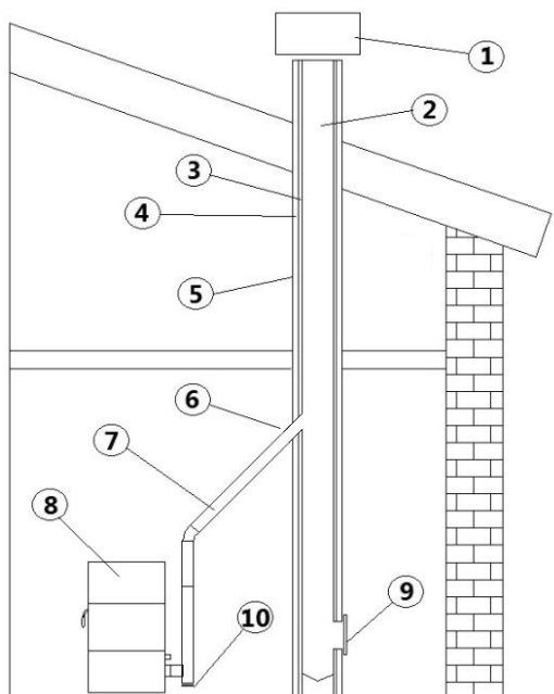
Fig. 6 - Części składowe komina
