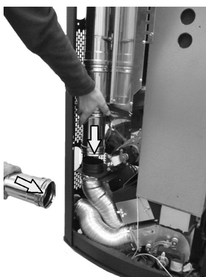
Fig. 63 - Układanie rur układu kanałowego
