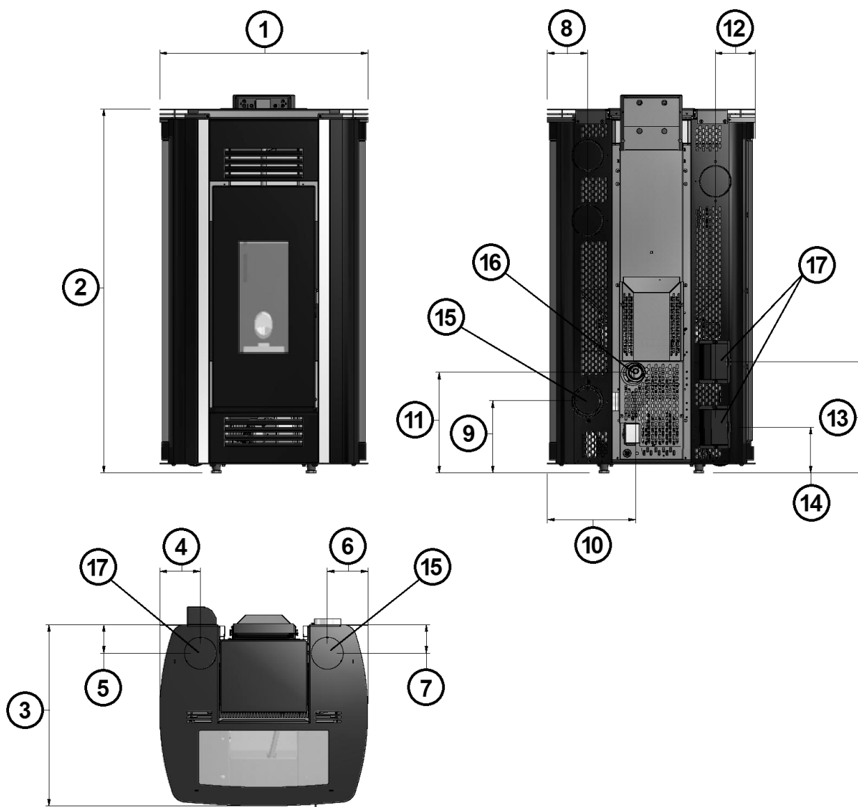
Fig. 21 - Ogólne wymiary: Venus 3 Plus 12,5KW
