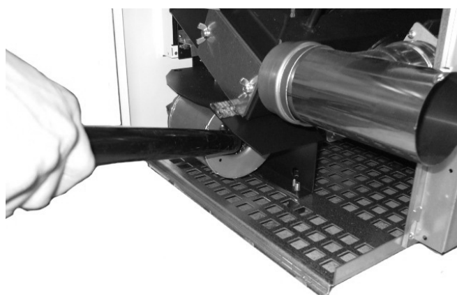
Fig. 107 - Czyszczenie wentylatora
