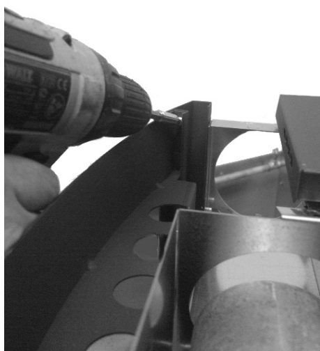
Fig. 44 - Usuwanie górnych zakrzywionych profili
