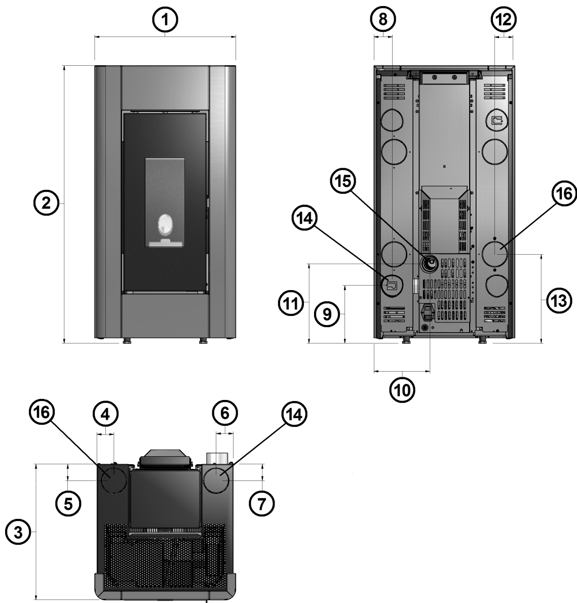
Fig. 19 - Ogólne wymiary: Prince 3 11KW / Prince 3 Plus 11KW
