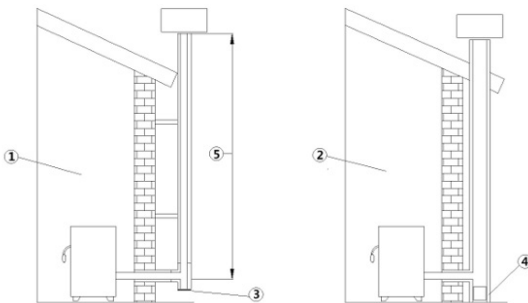
Fig. 2 - Kanały dymowe
