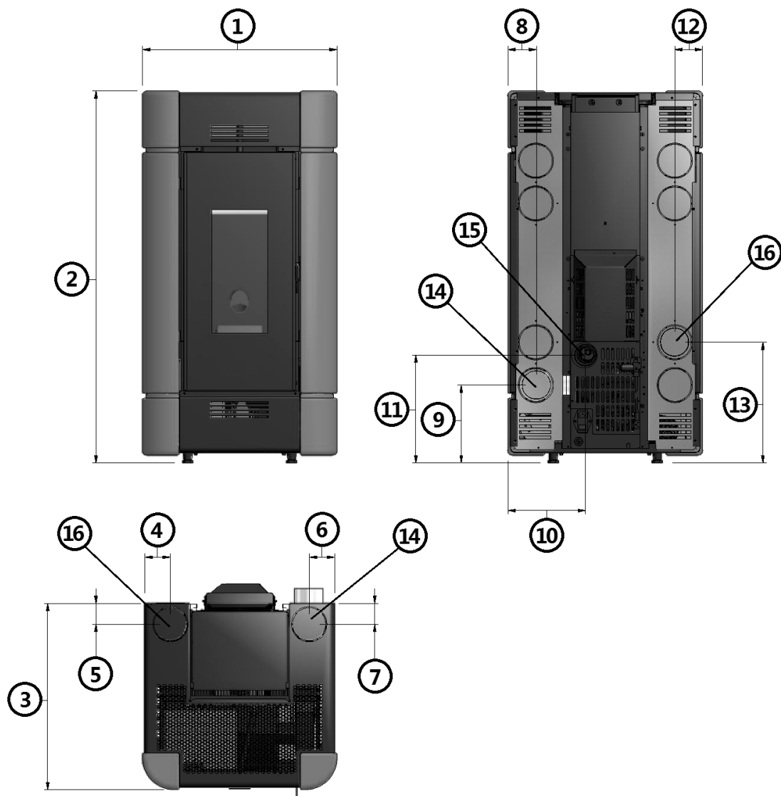
Fig. 16 - Ogólne wymiary: Sire 3 Plus 11KW
