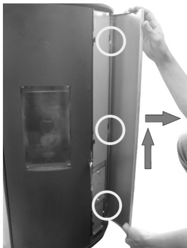
Fig. 36 - Montaż paneli
