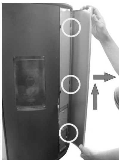
Fig. 80 - Sfera 3 / Sfera 3 Plus: odczepić panele boczne
