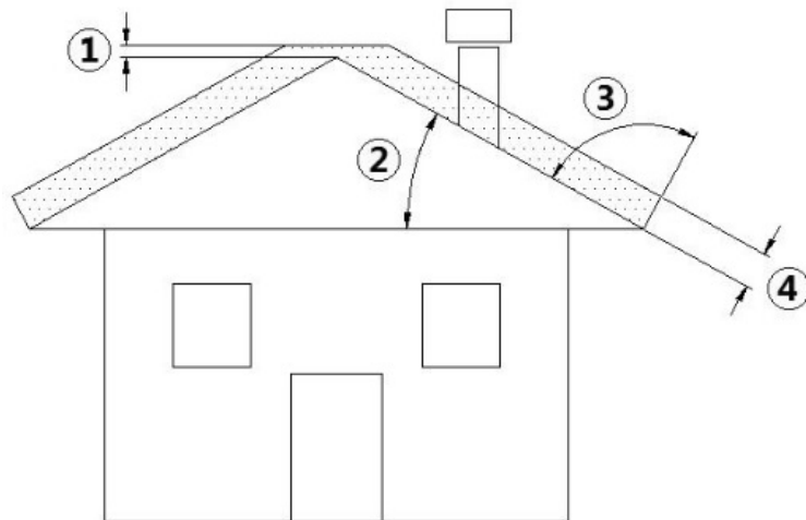
Fig. 3 - Dach skośny
