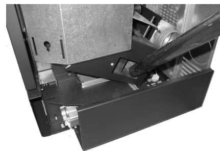
Fig. 101 - Czyszczenie komory dymu
