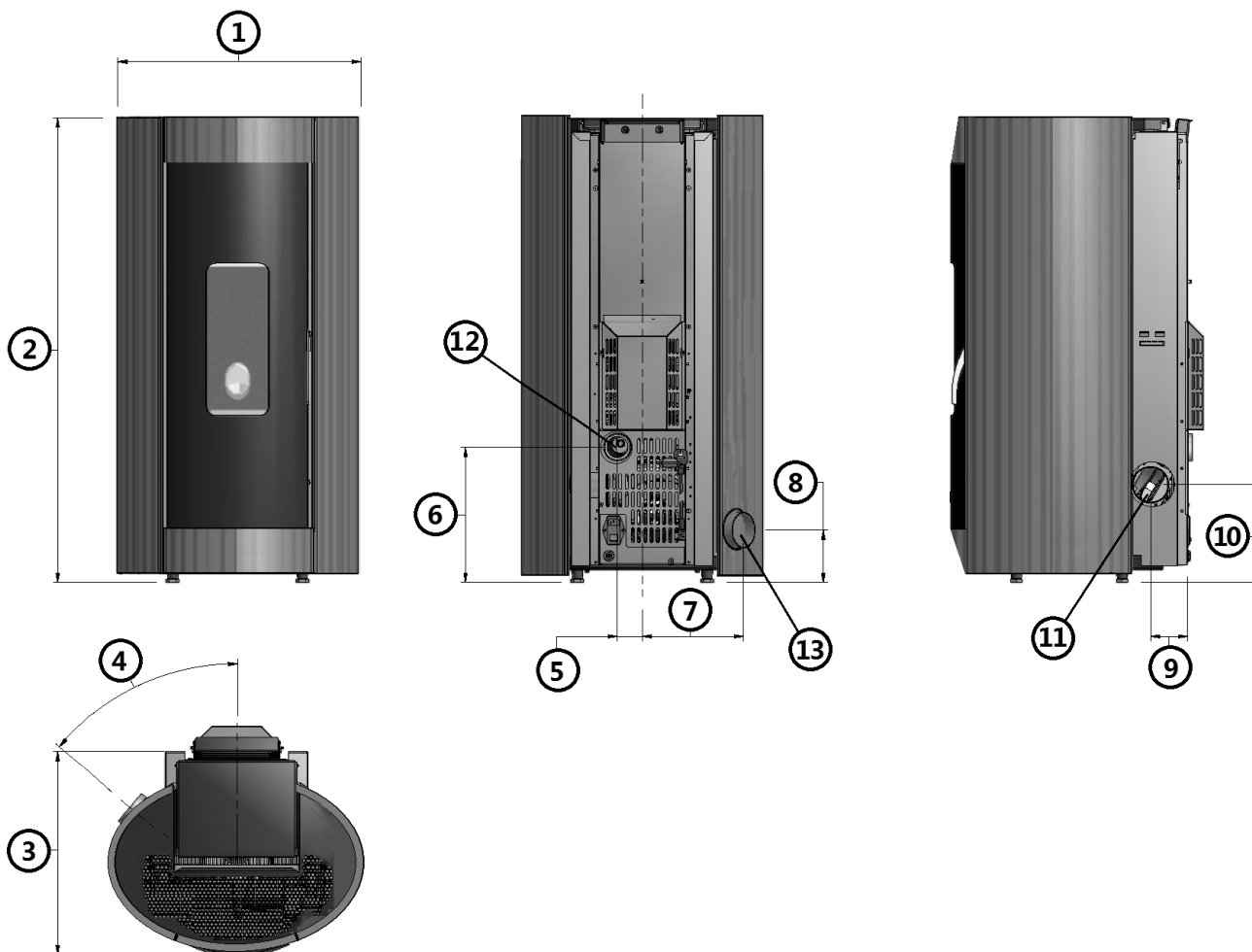
Fig. 20 - Ogólne wymiary: Elise³ Plus 11KW
