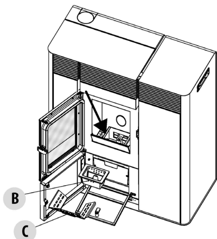
Fig. 20 - Wymywanie rusztu paleniskowego
