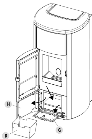
Fig. 18 - Wymywanie szuflady
