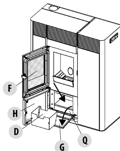
Fig. 21 - Wymywanie szuflady
