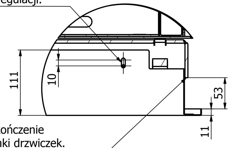
C (1 : 4)
