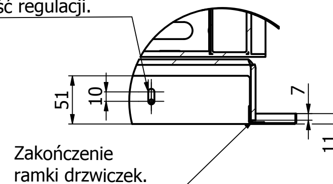
C ( 1 : 4 )
