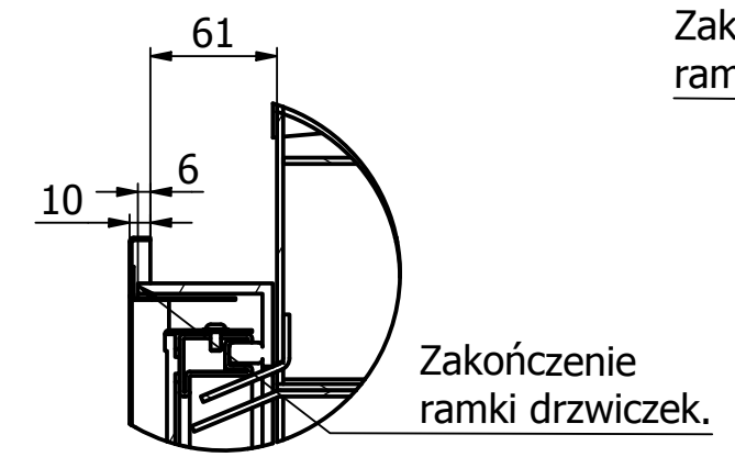
A ( 1 : 4 )
