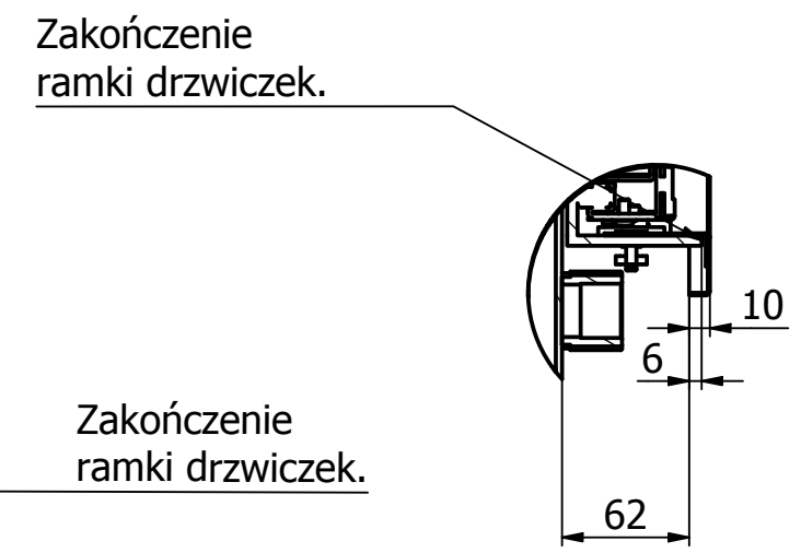
D ( 1 : 4 )
