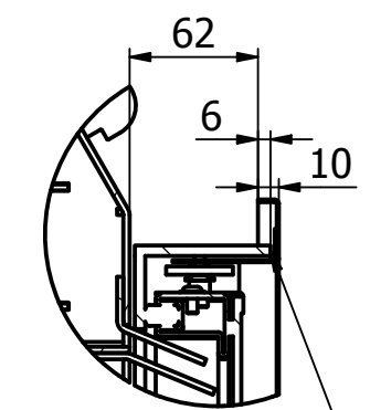
C ( 1 : 4 )
