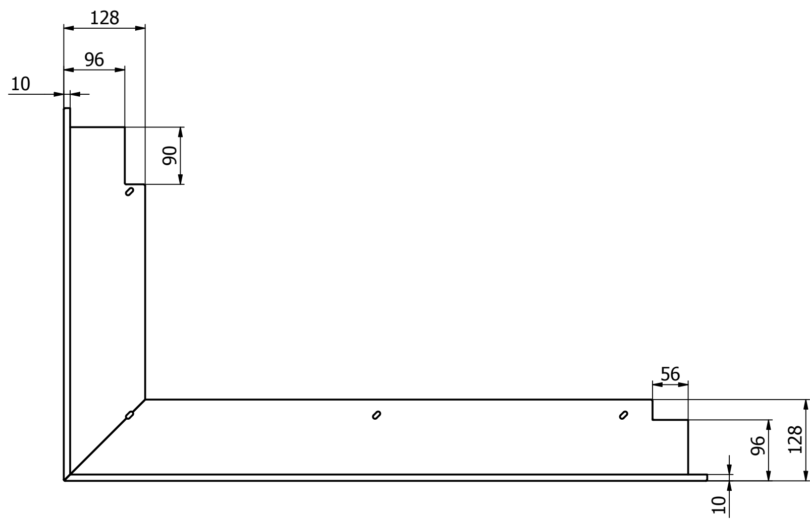
Maskownica 30 głęboka
