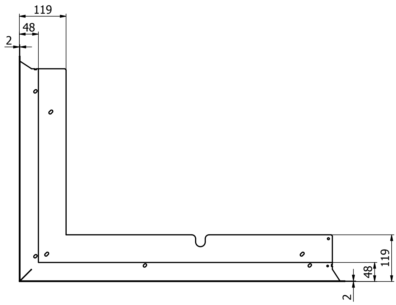
Maskownica kątowna płytka
