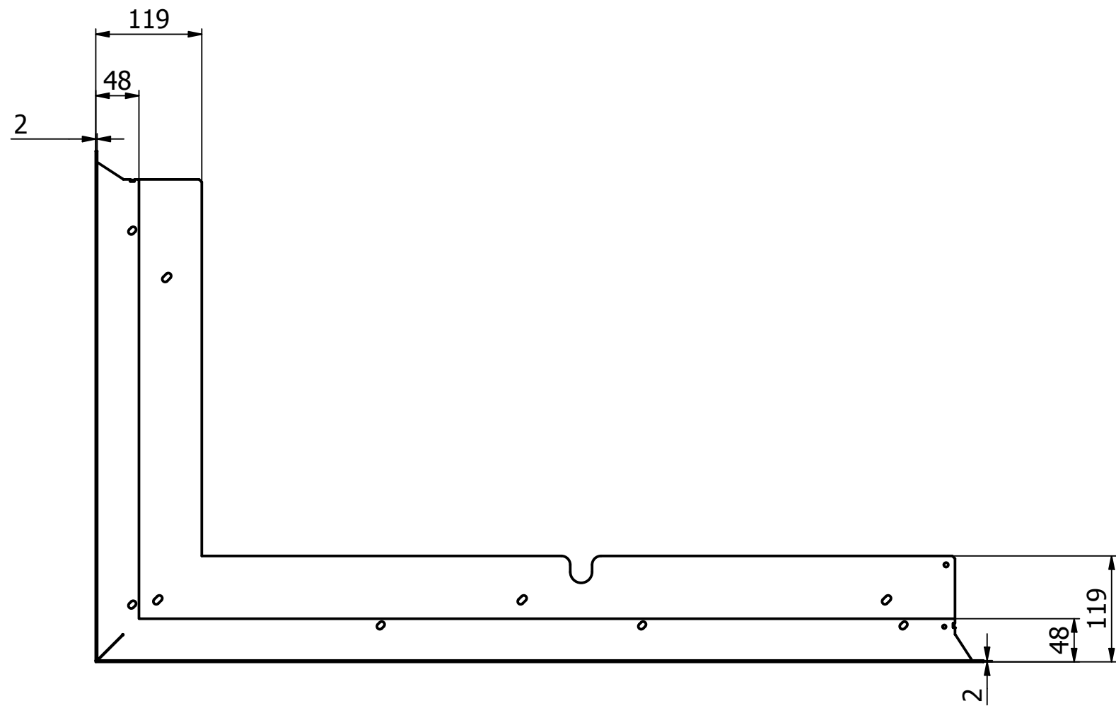
Maskownica kątowna płytka
