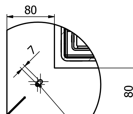
E (1 : 4)
