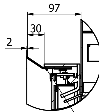
A (1 : 4)
