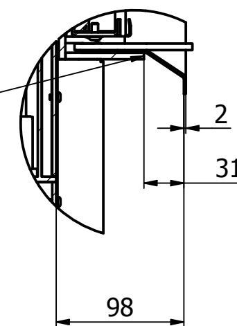
D (1 : 4)
