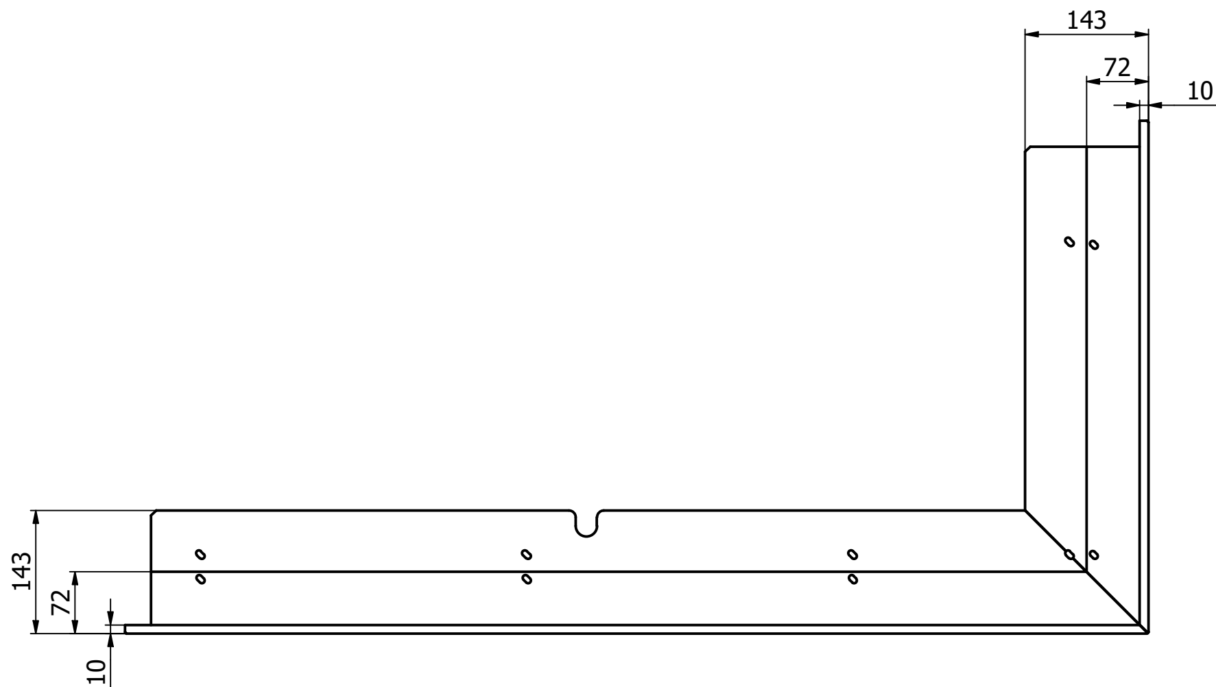
Maskownica 30 głęboka
