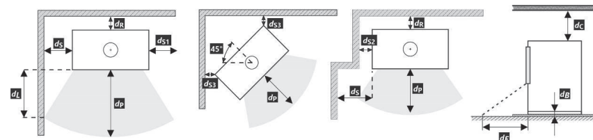
Rys. 2 Odległość od materiałów łatwopalnych
