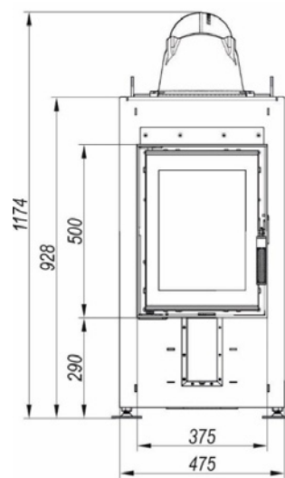
Vis XSM 6C MINI
