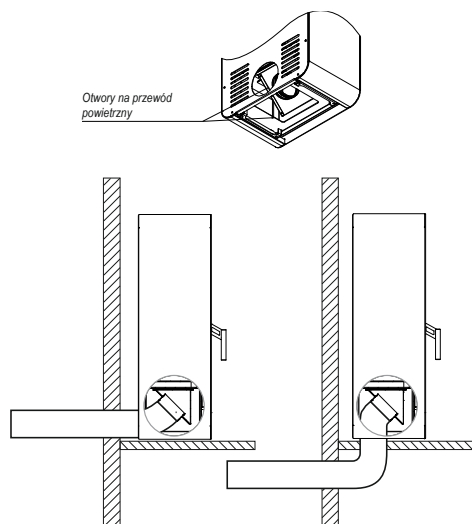
Rysunek 11. Podłączenie ogrzewacza serii DEFRO HOME PICO do zewnętrznego wlotu powietrza.
