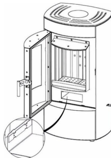
Krok 3. Kiedy zaślepka jest prawidłowo zamontowana należy wsunąć szufladę na popiół.
