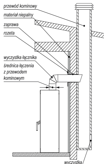
Rysunek 12. Podłączenie ogrzewacza kominkowego serii DEFRO HOME PICO do przewodu kominowego.
