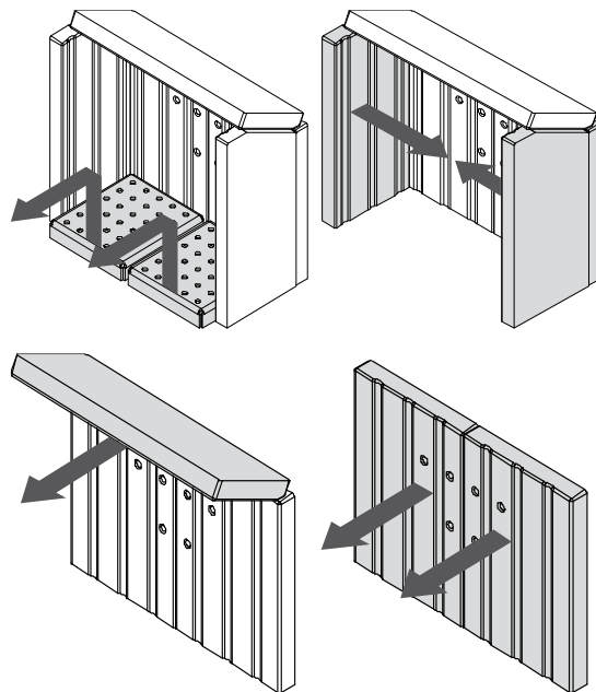
Rysunek 17. Kolejność demontażu płyt żaroodpornych komory paleniskowej.
