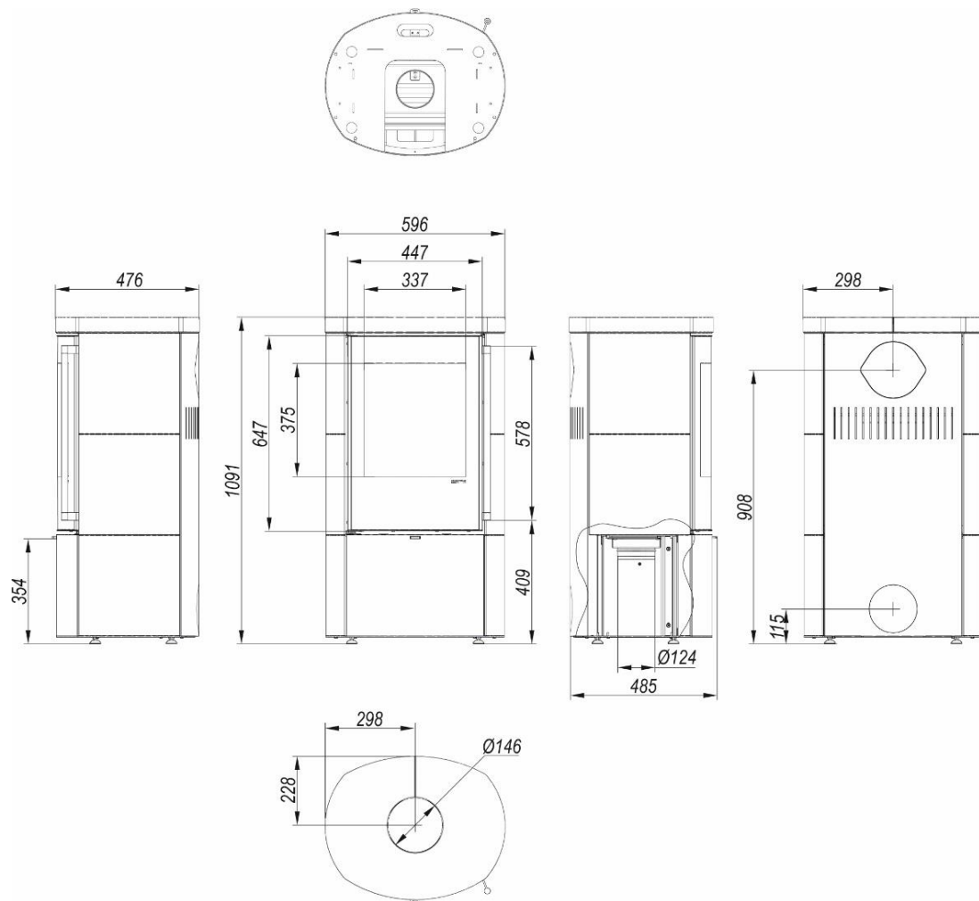
Rysunek 9. Wymiary (w mm) ogrzewacza DEFRO HOME CERES KRM
