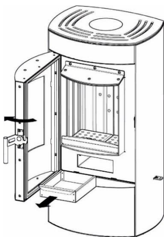
Krok 1. Otworzyć drzwi i wysunąć szufladę popielnika.
