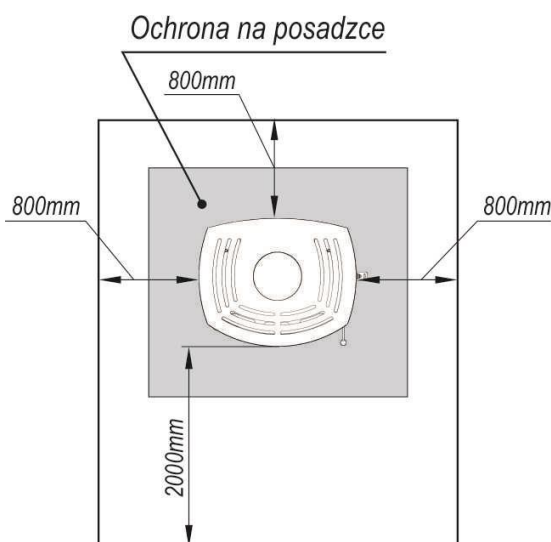
Rysunek 10. Minimalne bezpieczne odległości przy ustawianiu ogrzewacza.
