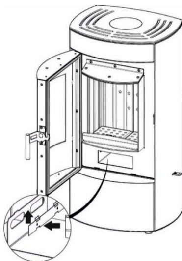
Krok 2. Po obu stronach komory popielnika zamontować zaślepki - Otworzyć drzwi i wysunąć szufladę popielnika. Wsunąć górne zatrzaski w wycięcia po bokach komory popielnika, a następnie dopchnąć dołem, tak aby zaślepka zatrzasknęła się. Należy zwrócić uwagę na doleganie zaślepki
