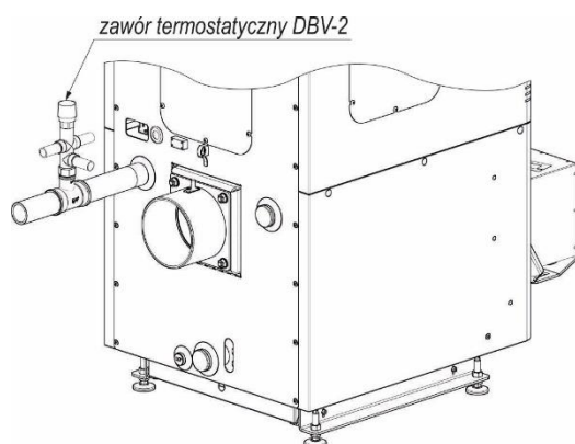
Rysunek 7. Sposób montażu zaworu termostatycznego DBV-2.
