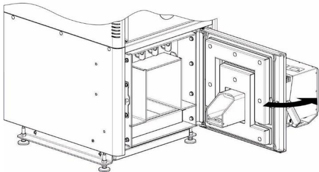
KROK 2. Otworzyć drzwi kotła.
