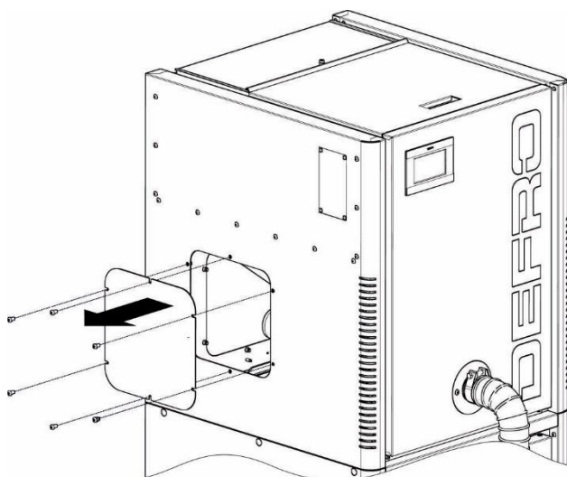
KROK 7. Odkręcić wkręty mocujące pokrywę rewizyjną i zdjąć pokrywę.
