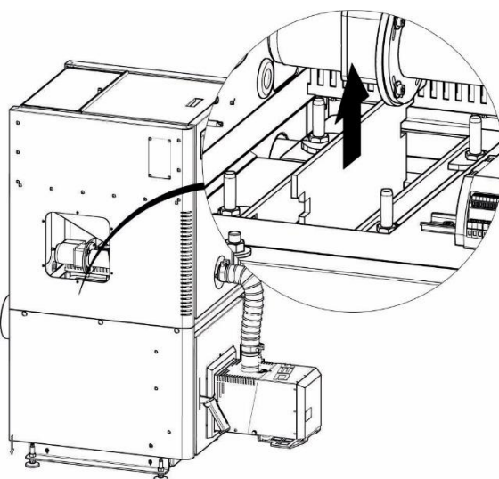
KROK 9. Wysunąć przegrodę kanału spalinowego i oczyścić. Oczyszczyć także ściany kanałów spalinowych.
