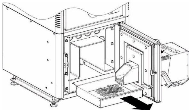
KROK 6. Usunąć nagromadzony popiół i pył
