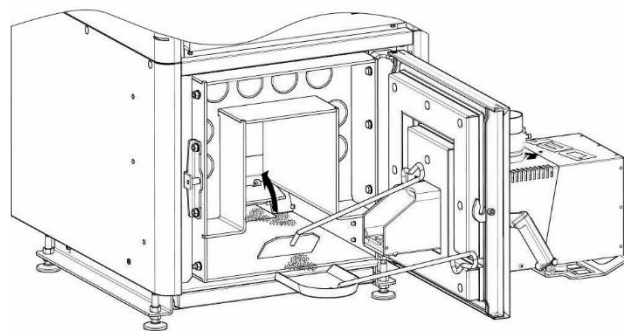
KROK 10. Po wysunięciu szuflady na popiół, odchylić klapę przegrody i wygarnąć nagromadzony popiół.
