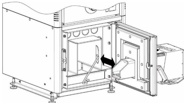
KROK 5. Za pomocą dostarczonych narzędzi oczyścić płomienicę
