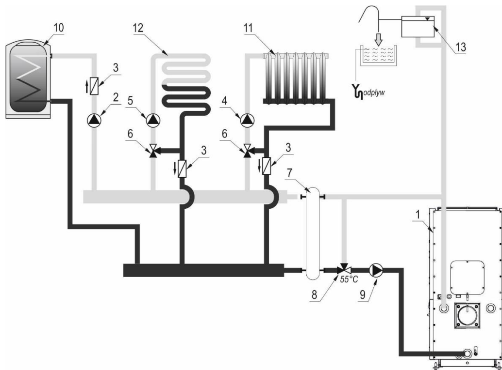
Rysunek 8. Uproszczony schemat instalacji grzewczej systemu otwartego.
