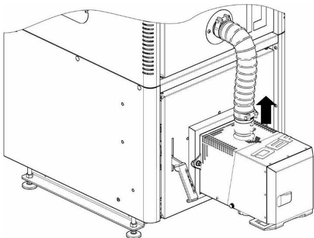
KROK 1. Zdemontować elastyczną rurę zsyłu paliwa.
