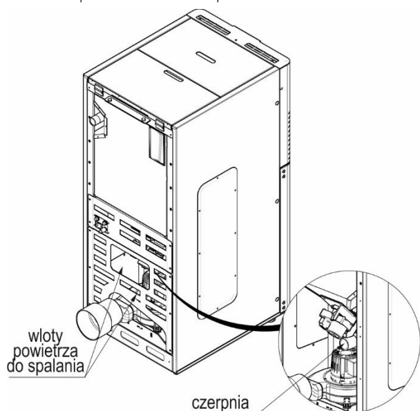
Rysunek 10. Czerpnia powietrza - otwór dolotowy powietrza.
