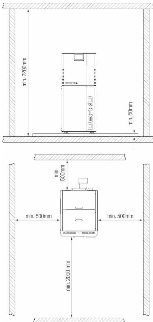
Rysunek 3. Ustawienie kotła w pomieszczeniu kotłowni.
