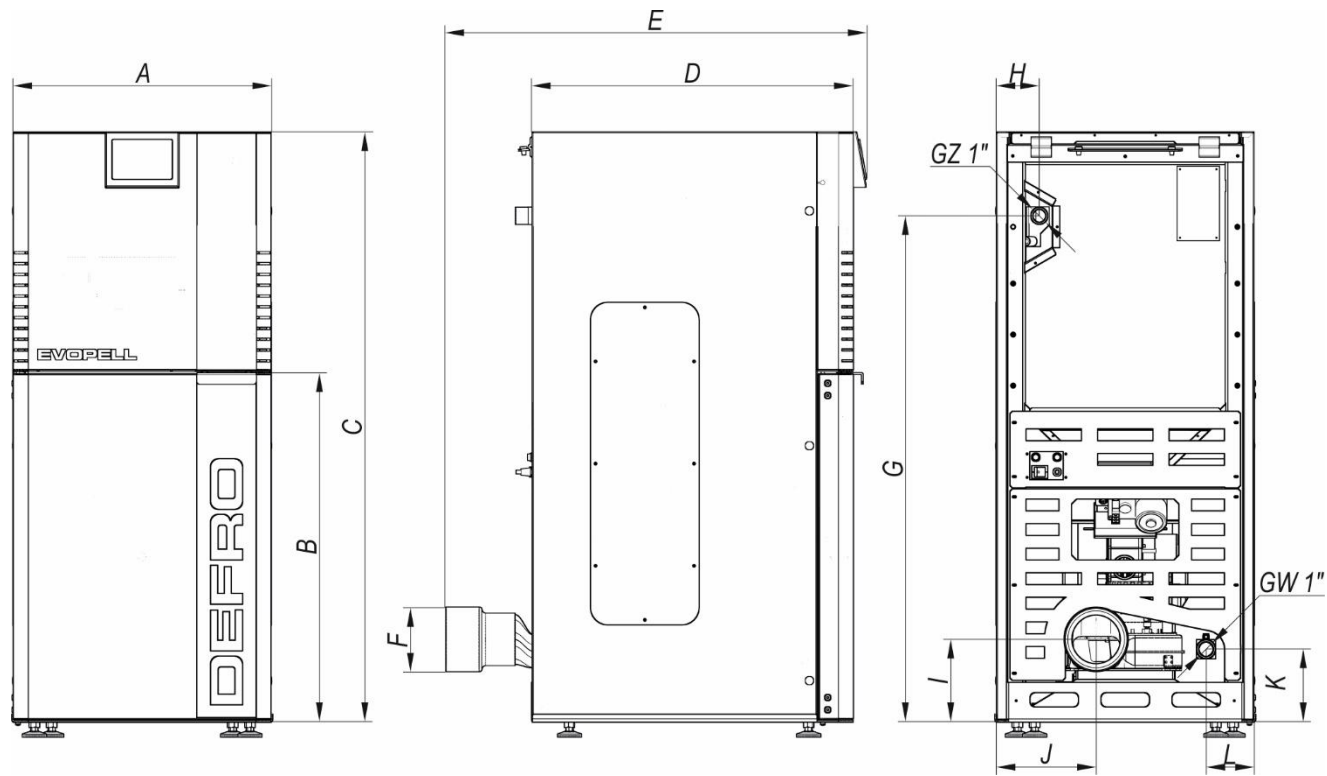
Rysunek 1. Podstawowe wymiary kotła.
