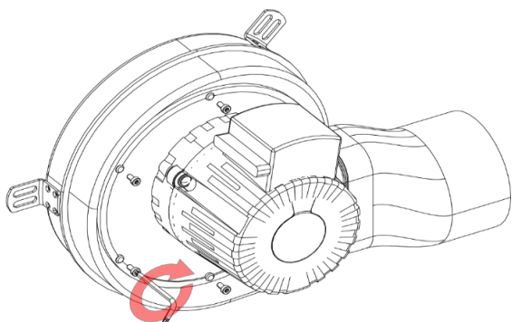
KROK 1. Odkręcić śruby mocujące wirnik wentylatora.
