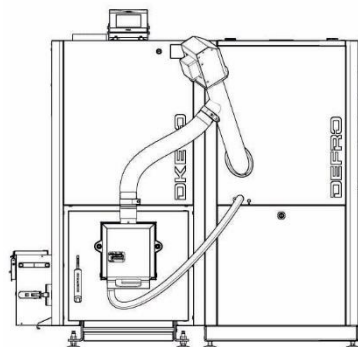
Rysunek 5. Prawidłowe połączenie rury podajnika.
