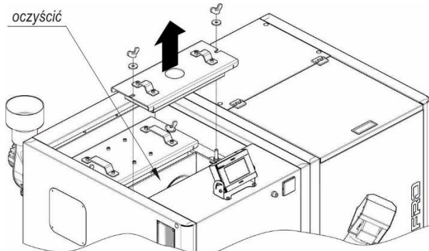
KROK 2. Odkręcić nakrętki mocujące pokrywę wyczystną i usunąć ją z kotła. Oczyszczyć ściany boczne wymiennika.
