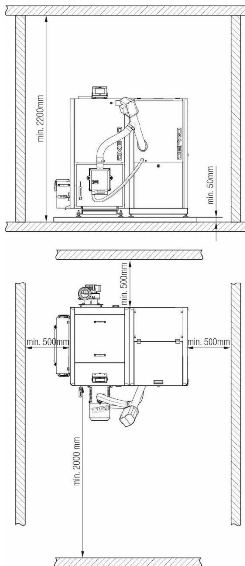
Rysunek 4. Ustawienie kotła w pomieszczeniu kotłowni.
