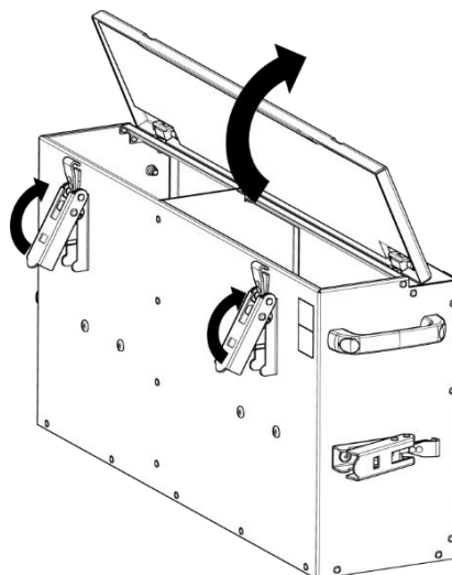
Rysunek 14. Sposób usuwania popiołu z zewnętrznego pojemnika.
