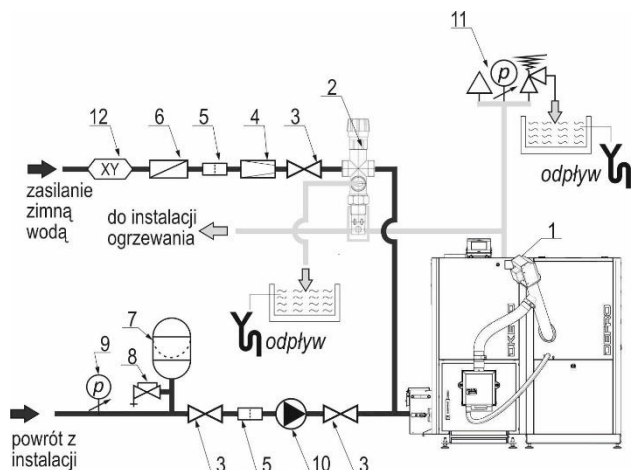
Rysunek 8. Przykładowy schemat zabezpieczeń kotła w układzie zamkniętym:
