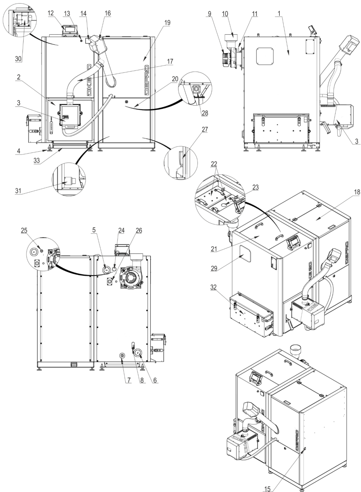
Rysunek 2. Podstawowe elementy kotła KOMPACT EKOPELL
