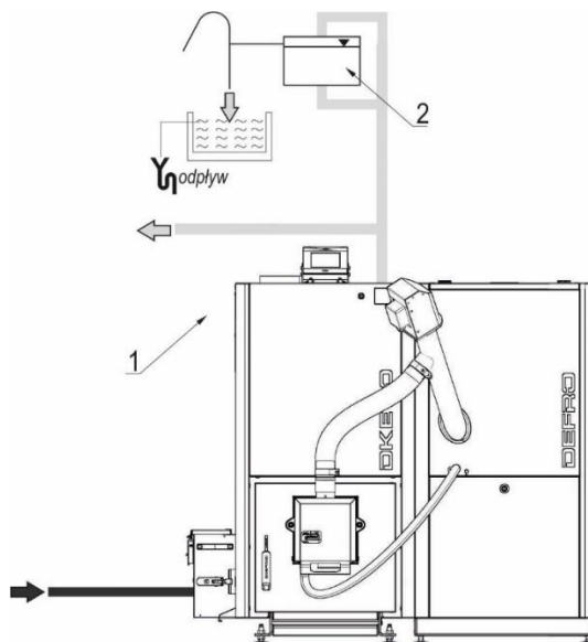
Rysunek 6. Przykładowy schemat zabezpieczeń kotła KOMPAKT EKO-PELL
