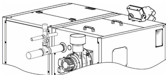
Rysunek 7. Przykładowy sposób podłączenia zaworu DBV-2.
