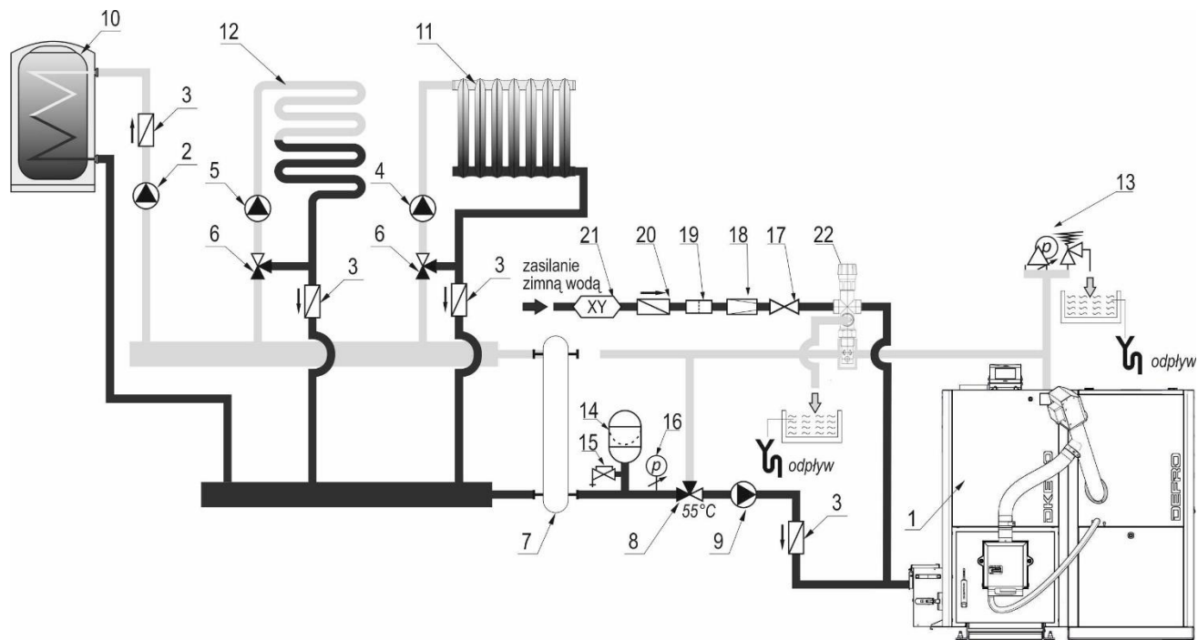
Rysunek 10. Uproszczony schemat instalacji grzewczej systemu zamkniętego.
