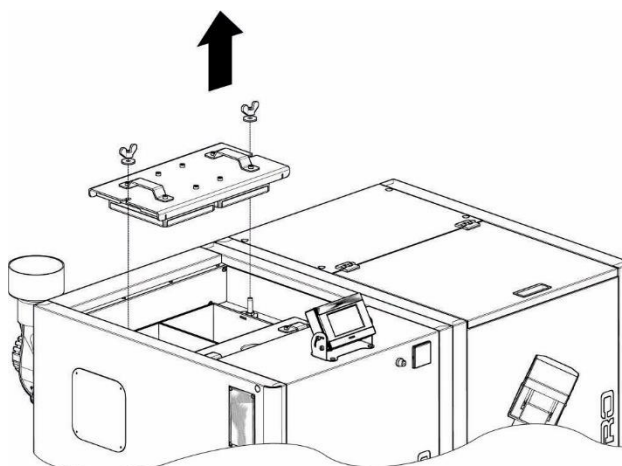
KROK 2. Odkręcić nakrętki mocujące pokrywę wyczystną i usunąć ją z kotła.
