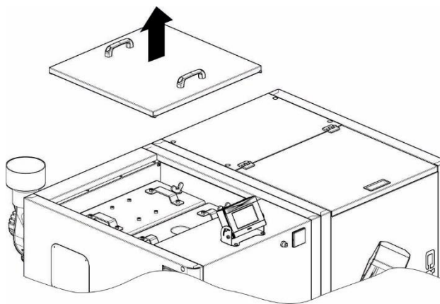
KROK 1. Podnieść pokrywę maskującą wyczystki górnej
