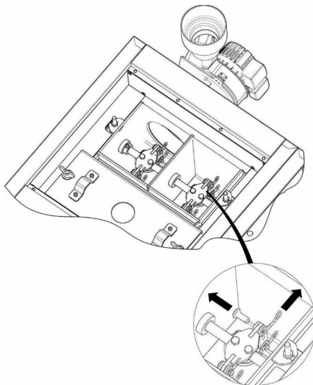
KROK 3. Wysunąć zawleczkę mocującą ramię mechanizmu, a następnie wysunąć trzpień.
