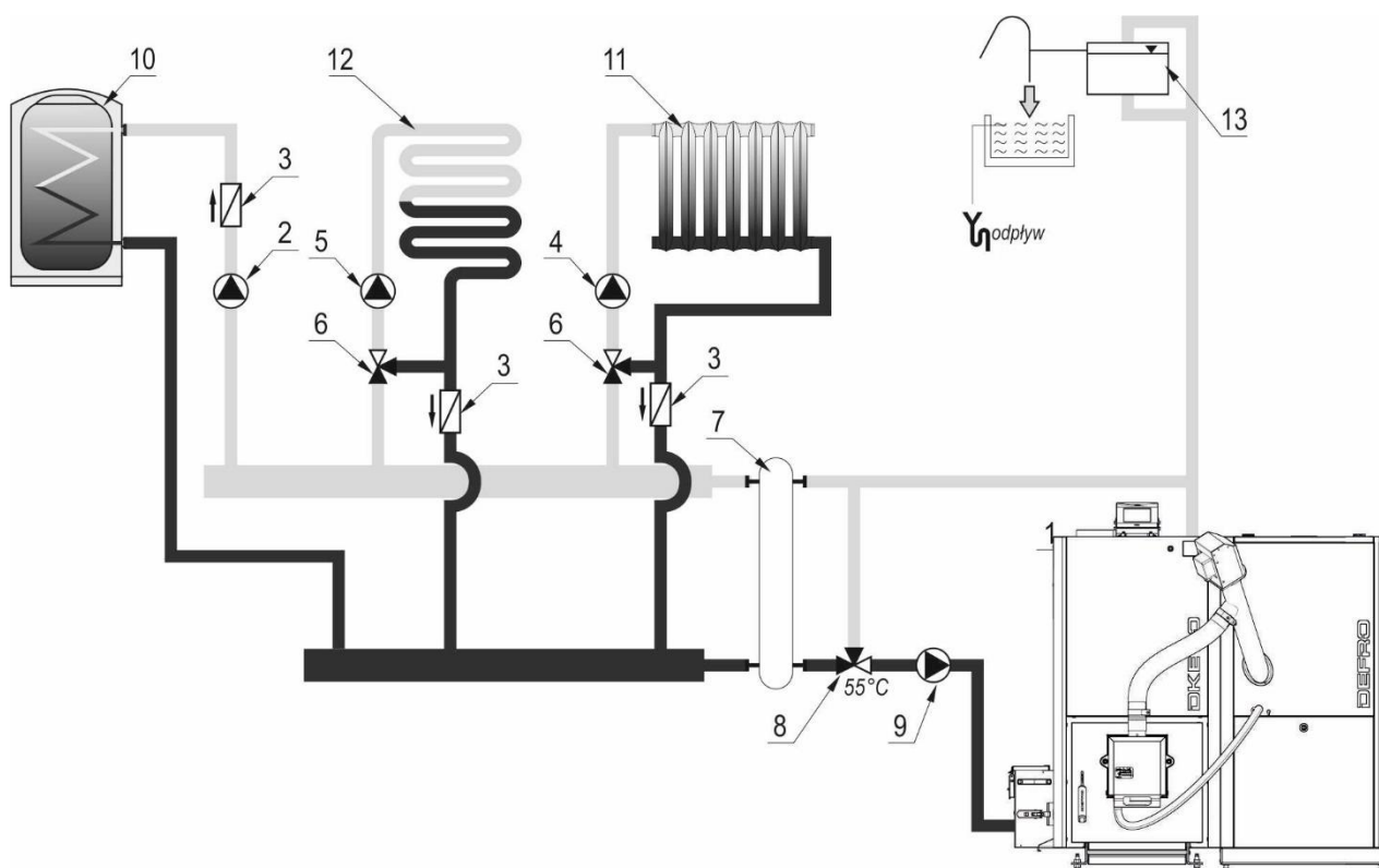
Rysunek 9. Uproszczony schemat instalacji grzewczej systemu otwartego.
