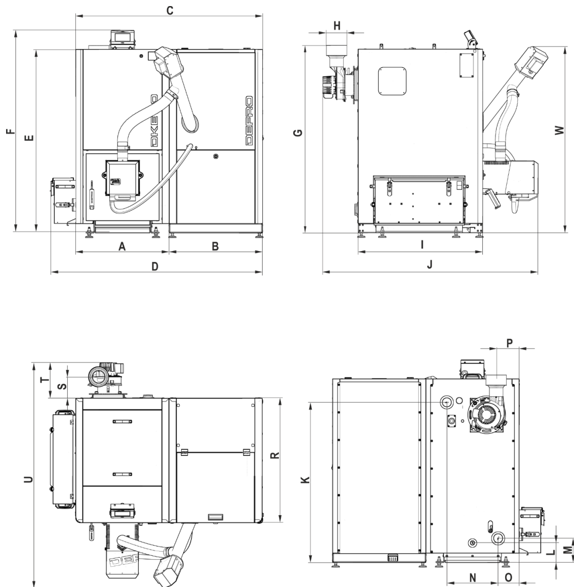
Rysunek 1. Podstawowe wymiary kotła KOMPAKT EKOPELL
