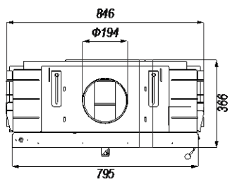
Rysunek 7. Wymiary wkładu kominkowego DEFRO HOME INTRA ME SLIM.
