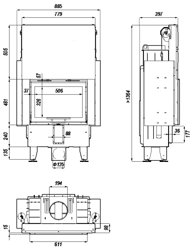
Rysunek 4. Wymiary wkładu kominkowego DEFRO HOME INTRA SM SLIM G.
