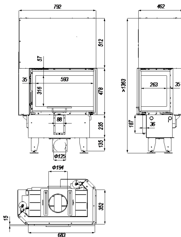
Rysunek 6. Wymiary wkładu kominkowego DEFRO HOME INTRA SM BP SLIM G.
