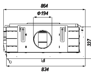
Rysunek 9. Wymiary wkładu kominkowego DEFRO HOME INTRA ME BP SLIM.
