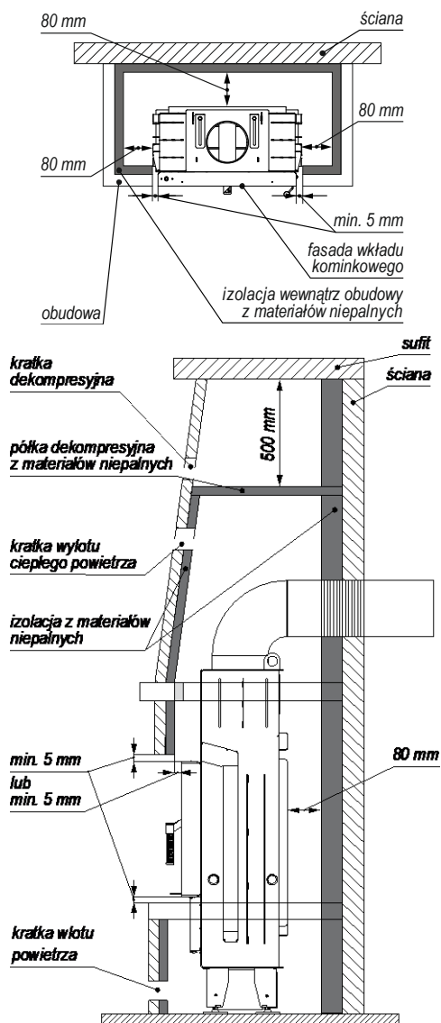
Rysunek 11. Przykładowa zabudowa wkładu kominkowego.
