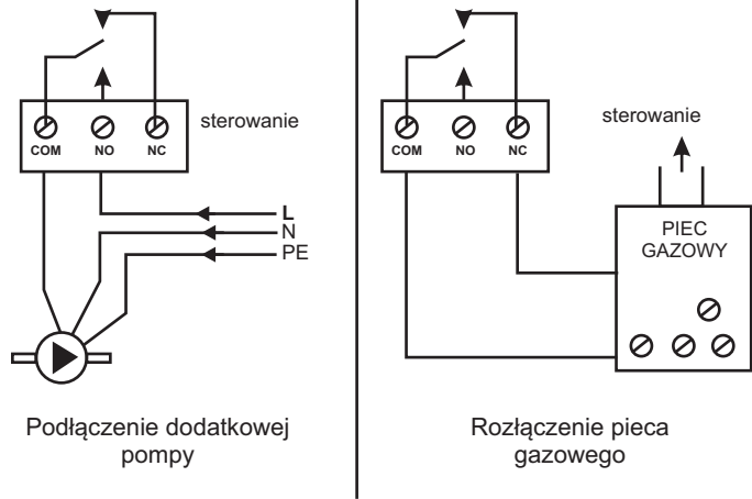
Rys.4 Schemat wykorzystania styku STEROWANIE
