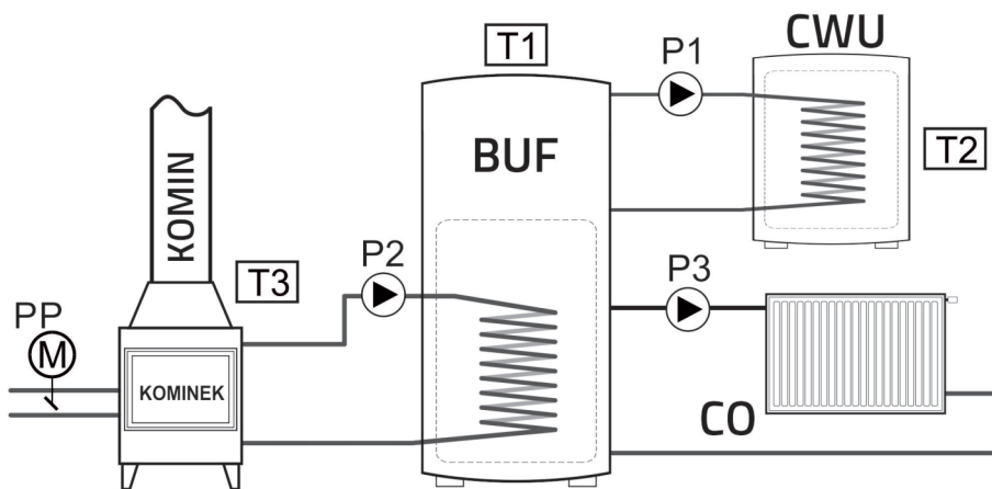
Rys.1a Podstawowy układ pracy regulatora (CWU za BUF).
