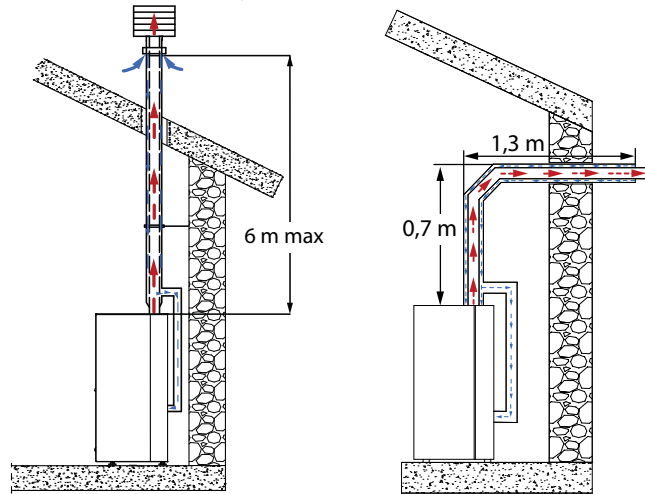
Instalacja współosiowa typu „e” i „f” z akcesoriami (jeśli są dołączone) *
