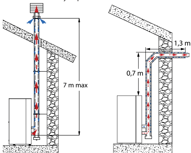
Instalacja współosiowa typu „c” i „d” (w stosownych przypadkach) *
