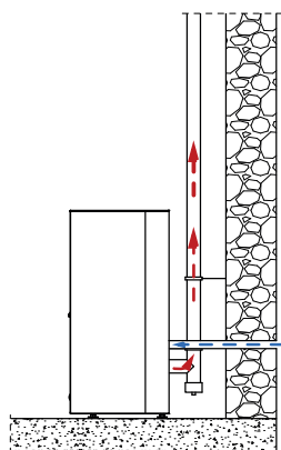
Typ instalacji „a”*
