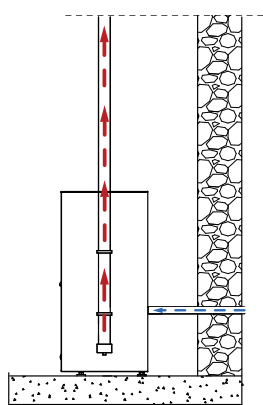
Typ instalacji „a”*
