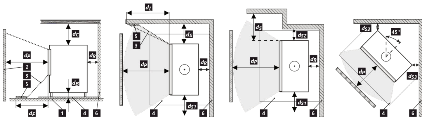
Rys. 2 Odległość od materiałów łatwopalnych
