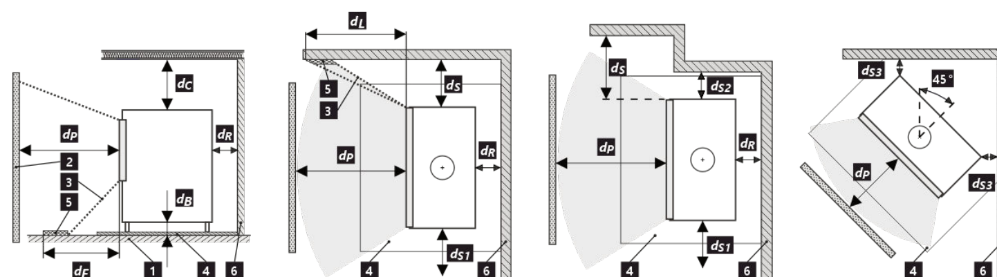
Obr. 2 Bezpečnostné odstupy od horľavých materiálov
