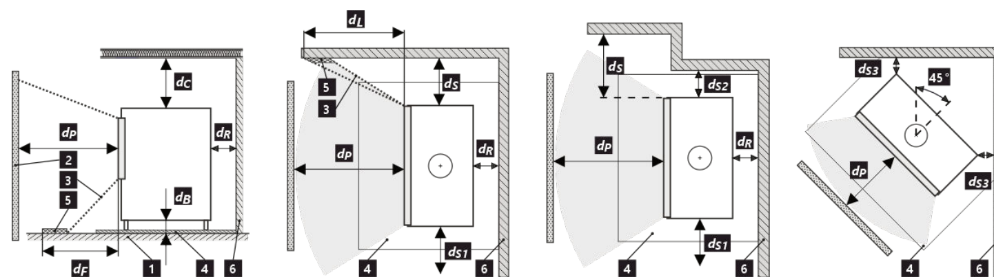
Kép 2 Távolság gyúlékony anyagoktól
