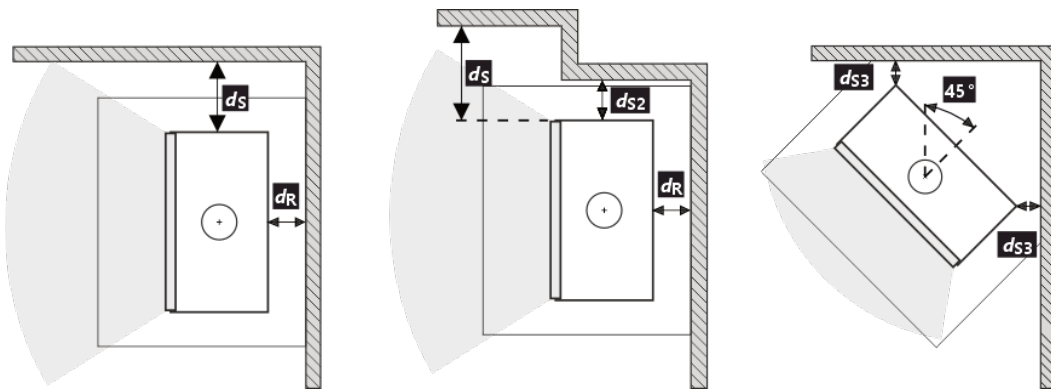
Kép 3. Távolság nem gyúlékony anyagoktól
