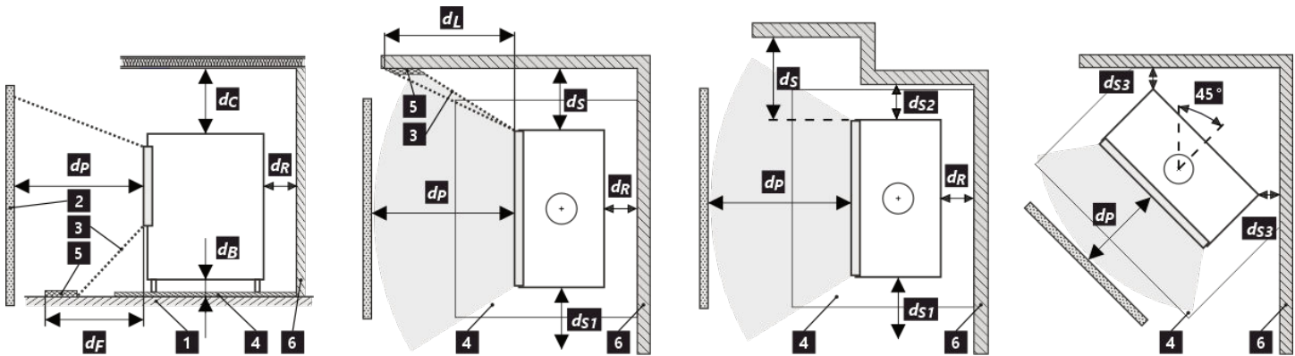
Рис. 2 Расстояние от горючих материалов
