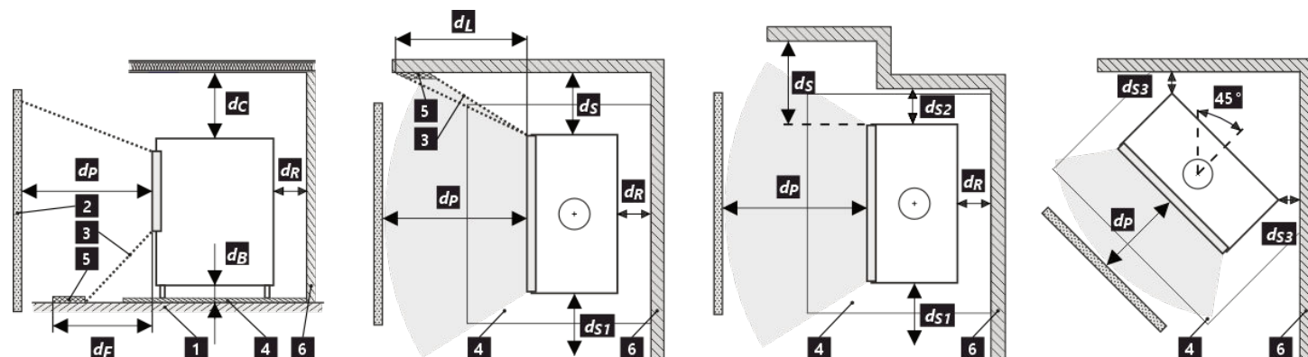
Obr. 2 Bezpečnostní odstupy od hořlavých materiálů
