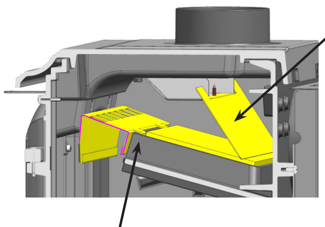
2 - DEFLEKTOR DYMU
