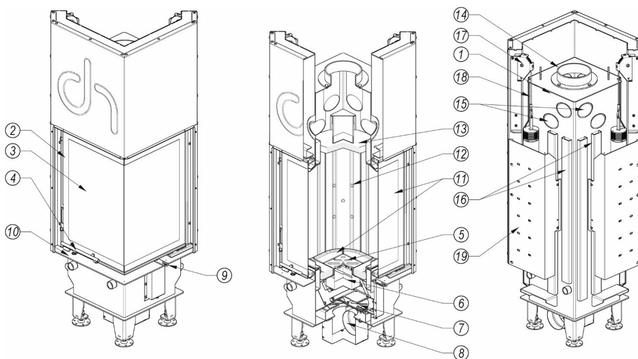
Rysunek 4. Budowa wkładu kominkowego DEFRO HOME INTRA I BP G
