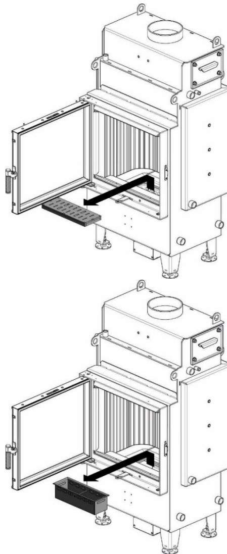
Rysunek 19. Wyjęcie rusztu i popielnika.
