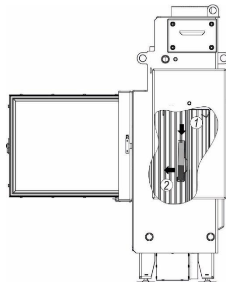
Rysunek 24. Sposób demontażu deflektowa
