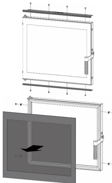
Rysunek 23. Demontaż szyby w drzwiach.
