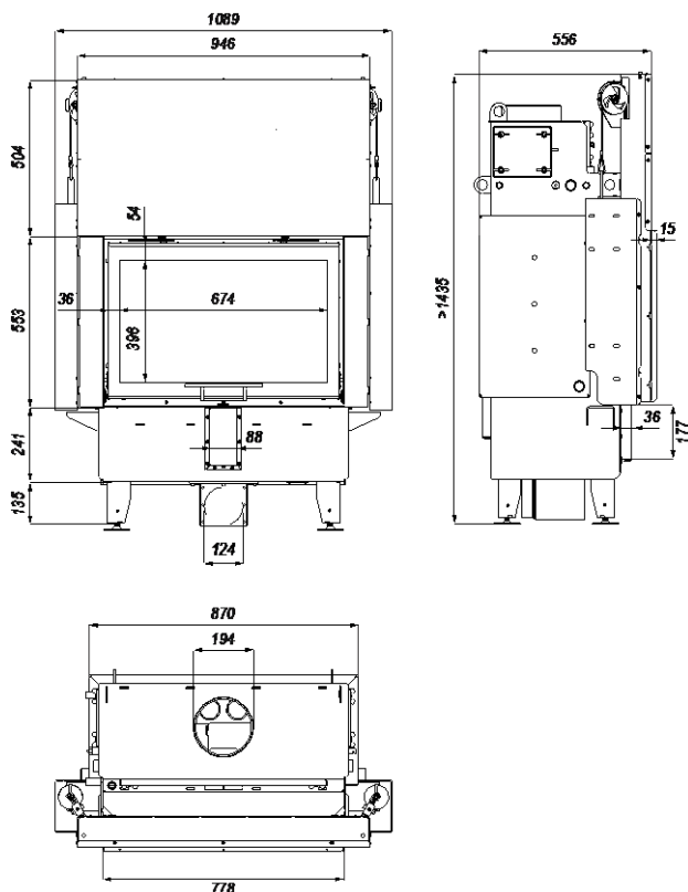
Rysunek 9. Rzuty z wymiarami wkładu kominkowego DEFRO HOME NAVI ME G
