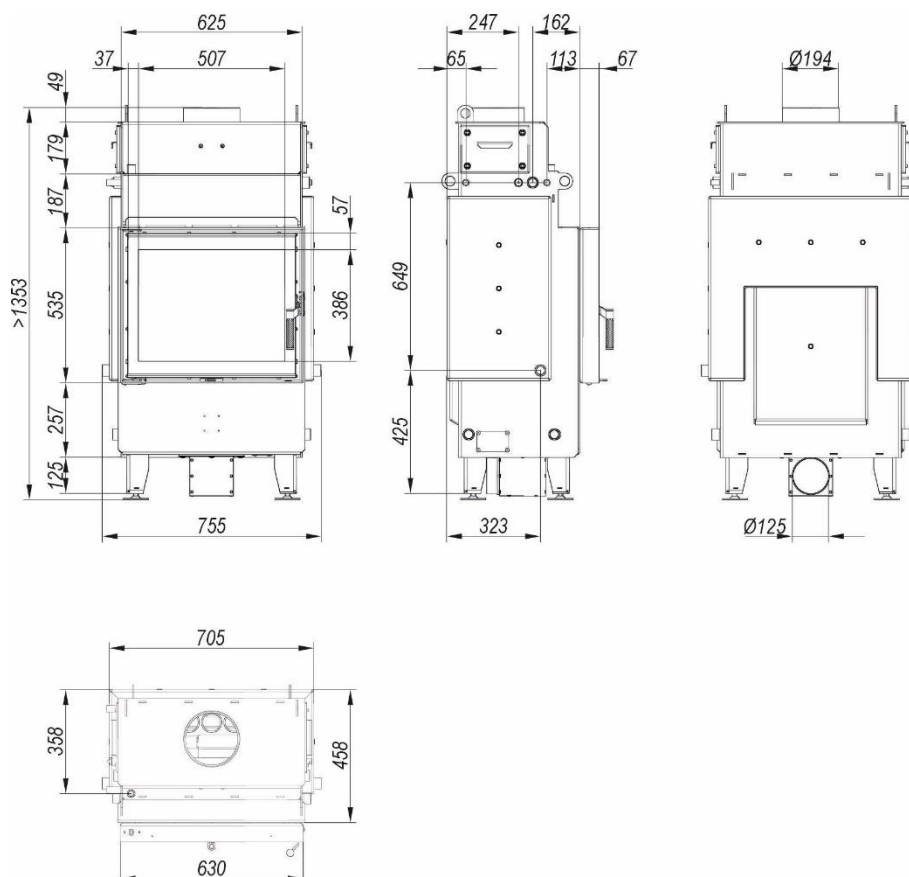
Rysunek 4. Rzuty z wymiarami wkładu kominkowego DEFRO HOME NAVI SM.
