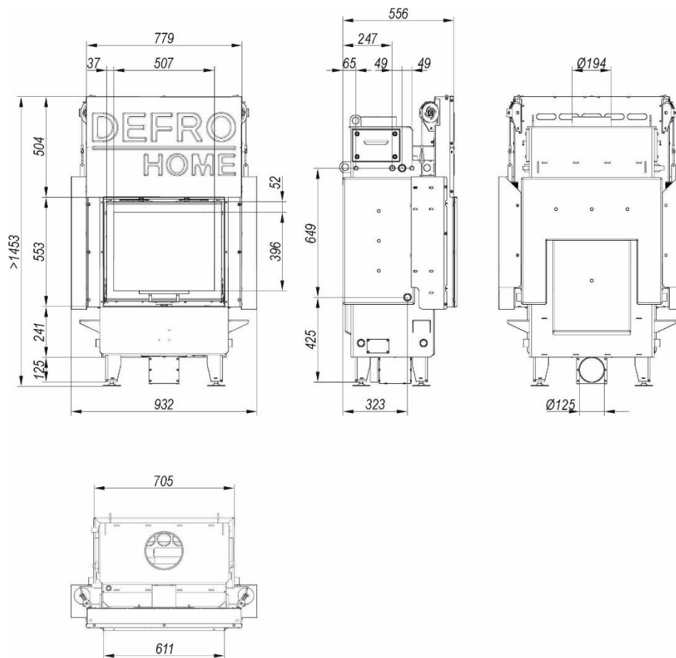
Rysunek 5. Rzuty z wymiarami wkładu kominkowego DEFRO HOME NAVI SM G.
