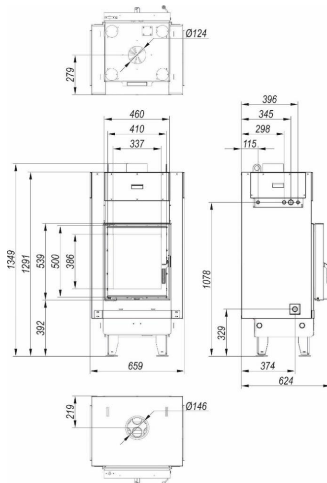
Rysunek 3. Rzuty z wymiarami wkładu kominkowego DEFRO HOME NAVI XSM w wersji z osłonami
