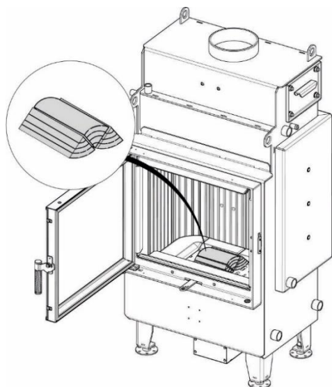
Rysunek 17. Sposób ułożenia paliwa (dla NAVI XSM -2 szczapy)
