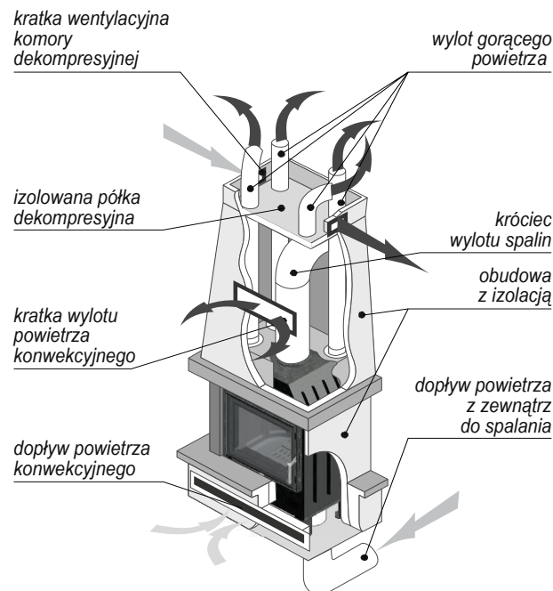
Rysunek 13. System dystrybucji gorącego powietrza.
