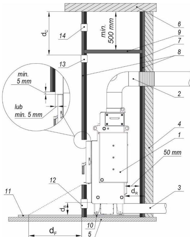
Rysunek 10. Przykładowa zabudowa wkładu kominkowego
