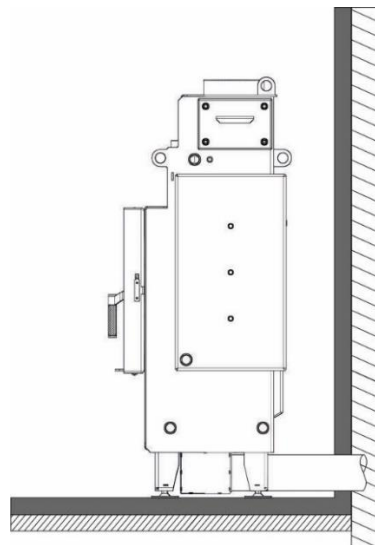
Rysunek 11. Podłączenie wkładu kominkowego do zewnętrznego wlotu powietrza.
