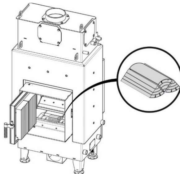
Rysunek 18. Sposób ułożenia paliwa w wersji DEFRO HOME NAVI TZ
