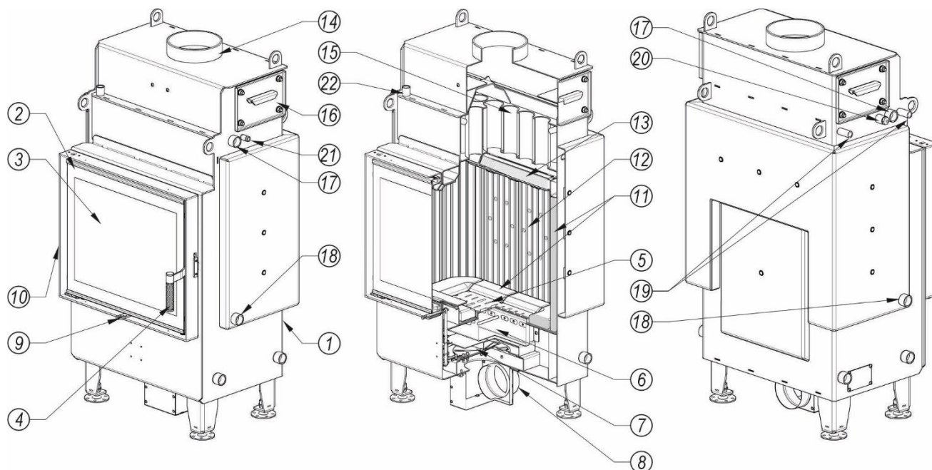
Rysunek 1. Budowa wkładu kominkowego DEFRO HOME NAVI z drzwiami rozwieralnymi.
