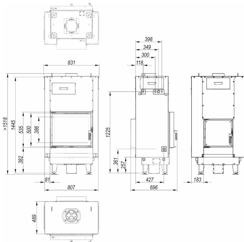
Rysunek 7. Rzuty z wymiarami wkładu kominkowego DEFRO HOME NAVI SM TZ w wersji z osłonami
