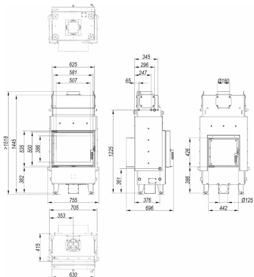
Rysunek 6. Rzuty z wymiarami wkładu kominkowego DEFRO HOME NAVI SM TZ
