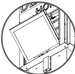
Rysunek 21. Widok drzwi wkładu DEFRO HOME NAVI G w pozycji uchylnej.
