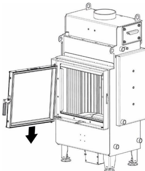
Rysunek 22. Sposób demontażu drzwi wkładu kominkowego
