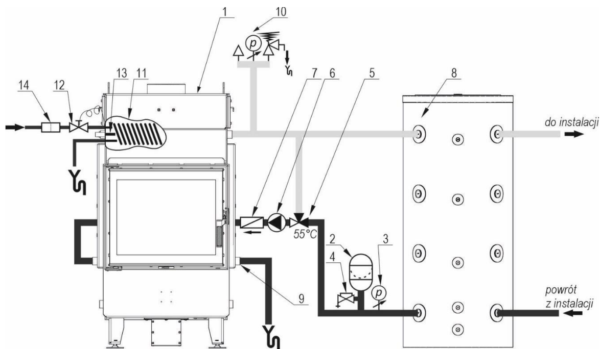
Rysunek 15. Schemat przykładowego podłączenia zespołu wodnego kominka DEFRO HOME NAVI z systemem grzewczym w układzie zamkniętym.
