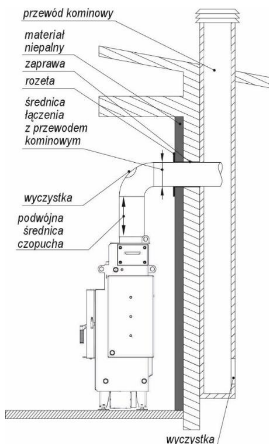
Rysunek 12. Podłączenie wkładu kominkowego do przewodu kominowego.
