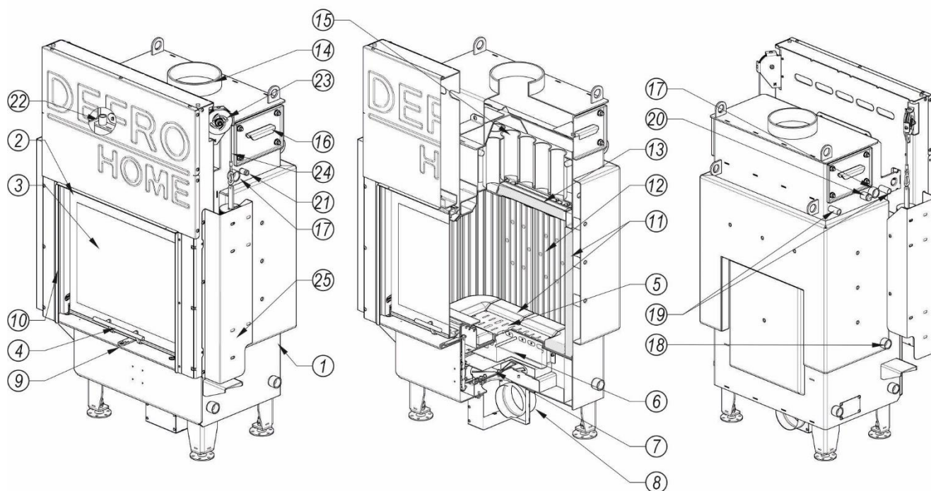
Rysunek 2. Budowa wkładu kominkowego DEFRO HOME NAVI G z drzwiami podnoszonymi
