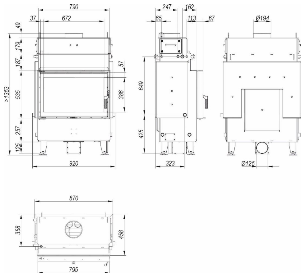
Rysunek 8. Rzuty z wymiarami wkładu kominkowego DEFRO HOME NAVI ME.
