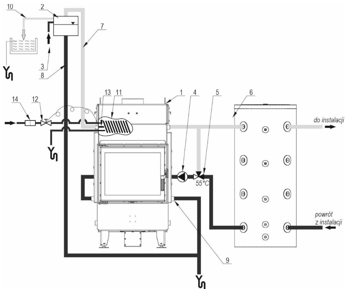
Rysunek 14. Schemat przykładowego podłączenia zespołu wodnego kominka DEFRO HOME NAVI z systemem grzewczym w układzie otwartym.
