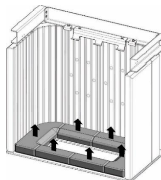
Rysunek 24. Sposób demontażu deflektowa
