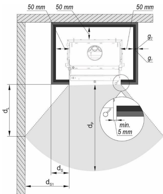
Rysunek 10. Przykładowa zabudowa wkładu kominkowego
