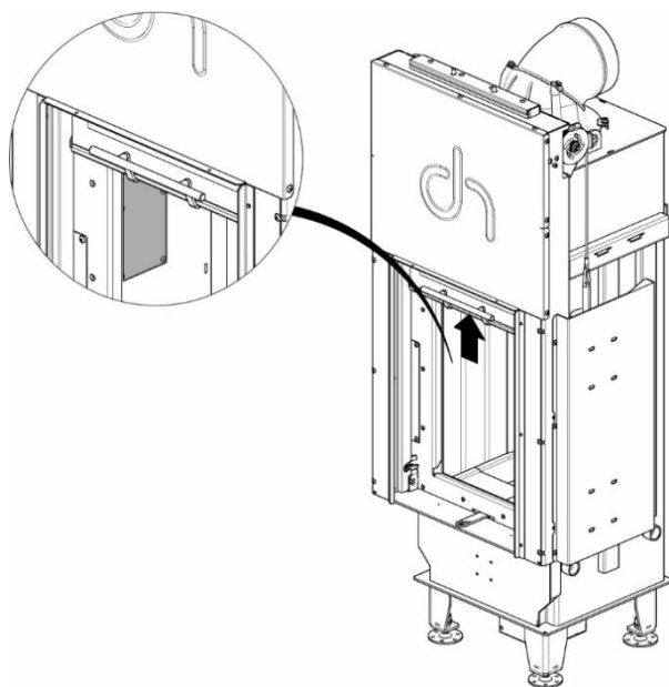
Rysunek 23. Umieszczenie pokryw otworów rewizyjnych we wkładzie: DEFRO HOME INTRA I wersja G.
