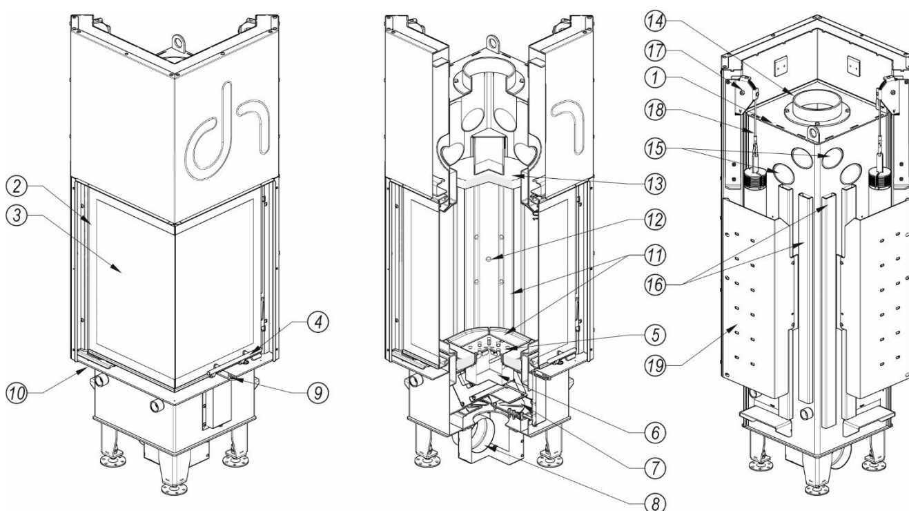
Rysunek 4. Budowa wkładu kominkowego DEFRO HOME INTRA I BL G
