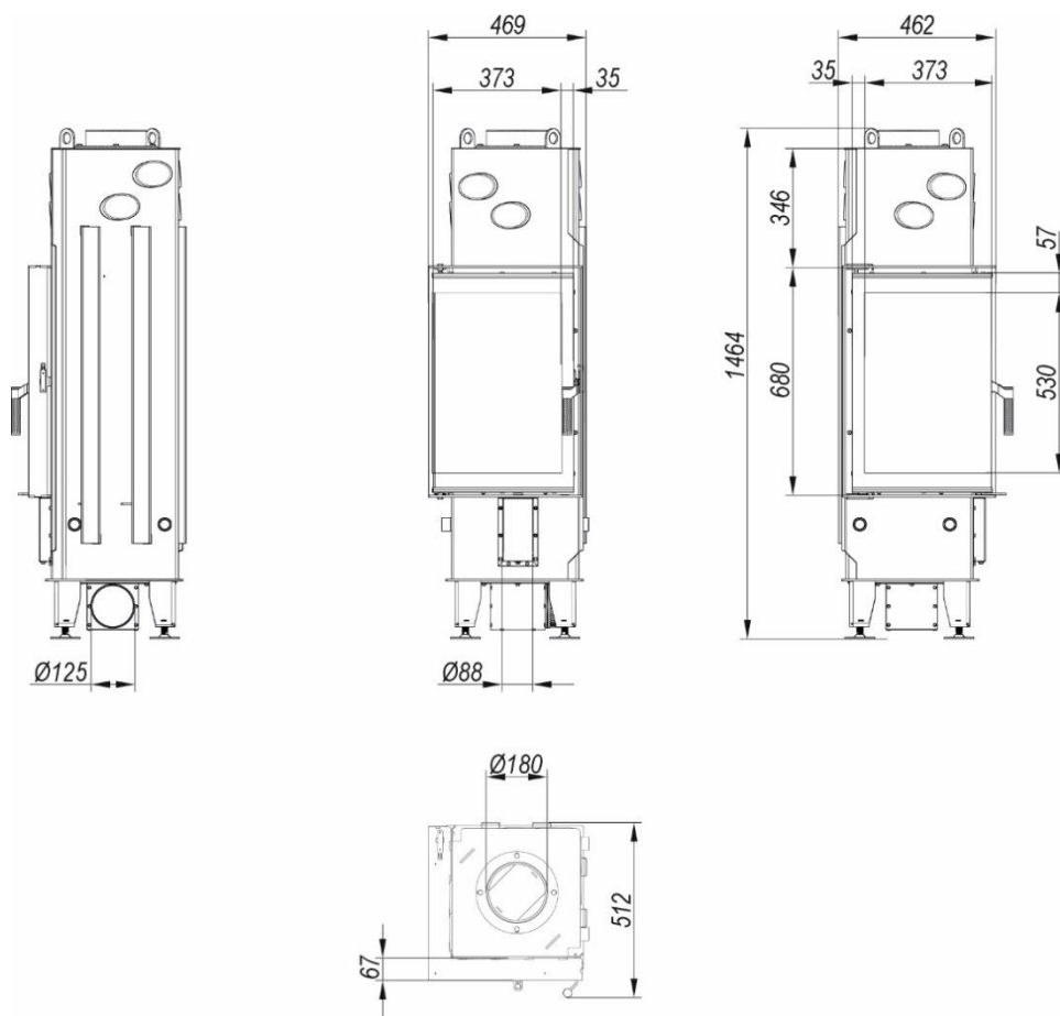
Rysunek 7. Wymiary wkładu kominkowego DEFRO HOME INTRA I BL
