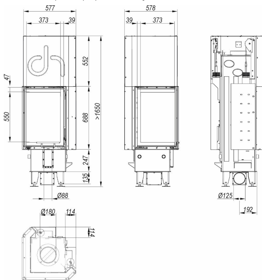
Rysunek 8. Wymiary wkładu kominkowego DEFRO HOME INTRA I BL G
