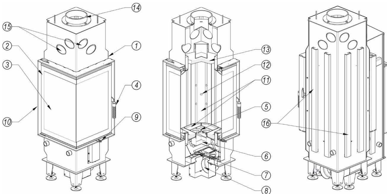
Rysunek 3. Budowa wkładu kominkowego DEFRO HOME INTRA I BL
