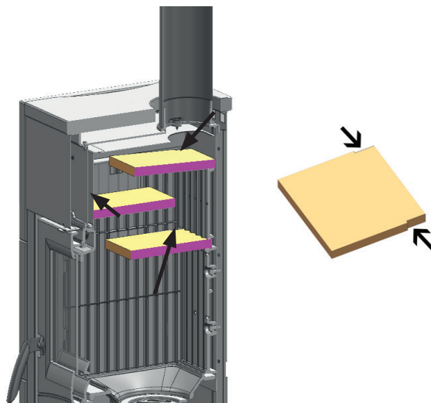
2 - DEFLEKTOR DYMU
