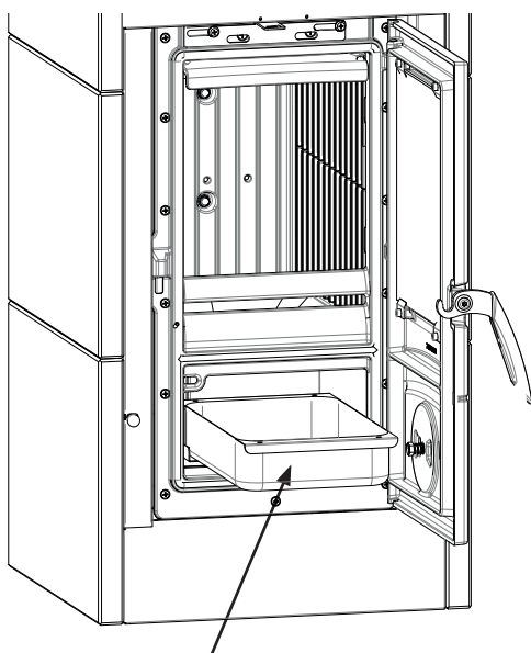
1 - SZUFLADA NA POPIÓŁ
