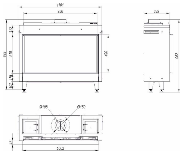
Rysunek 15. Wymiary DEFRO HOME VITAL 51 M.
