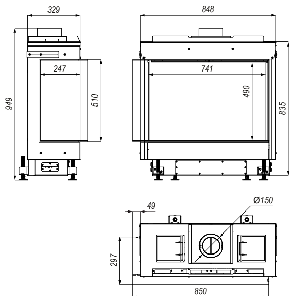
Rysunek 10. Wymiary DEFRO HOME VITAL 51 S BL i DEFRO HOME VITAL 51 S BP (odbicie lustrzane).
