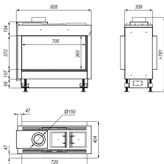
Rysunek 5. Wymiary DEFRO HOME VITAL 37 S T
