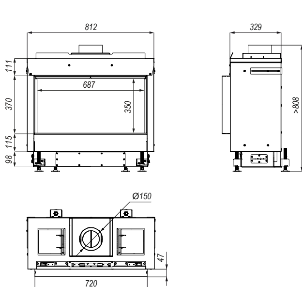
Rysunek 2. Wymiary DEFRO HOME VITAL 37 S.
