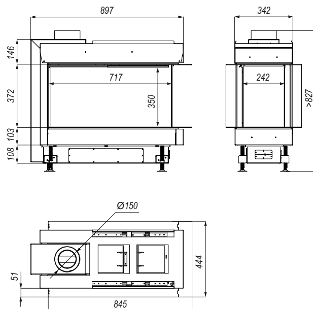
Rysunek 7. Wymiary DEFRO HOME VITAL 51 S U.
