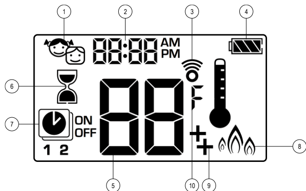
Rysunek 29. Ekran wyświetlacza pilota.
