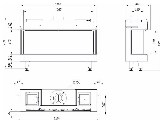
Rysunek 13. Wymiary DEFRO HOME VITAL 37 M C.
